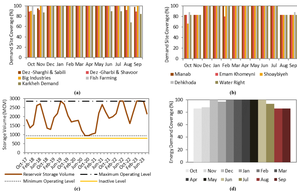
شکل ۷. نتایج اجرای سناریوی دوم: a- متوسط درصد تأمین نیاز مصارف بالادست منطقه مطالعاتی دز b- متوسط درصد تأمین نیاز مصارف پایین دست منطقه مطالعاتی c- تغییرات حجم ذخیره ماهانه مخزن سد در طول دوره بهره‌برداری ۶ ساله d- متوسط درصد تأمین نیاز برق تولیدی
