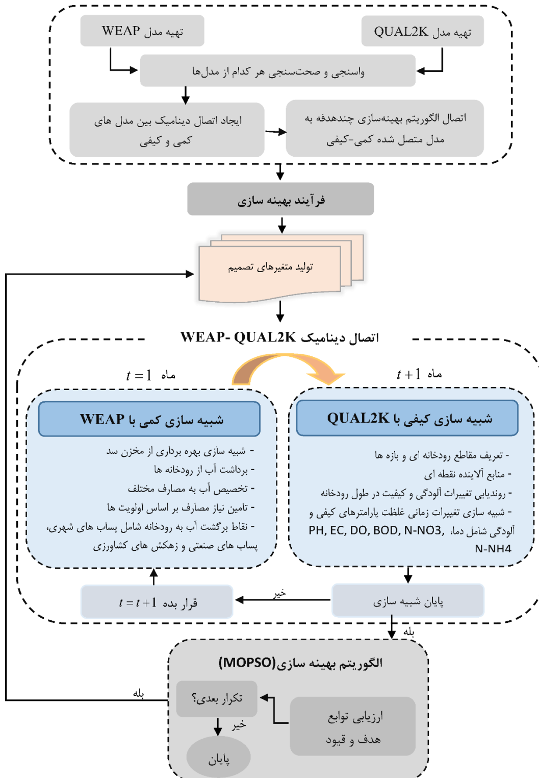
شکل ۱. ساختار مدل کوپل شده شبیه‌سازی-بهینه‌سازی
