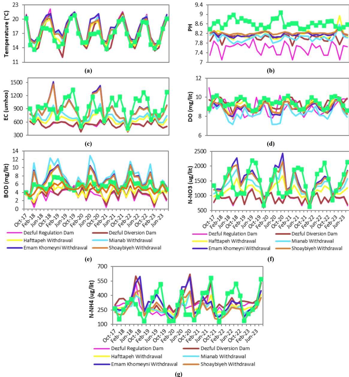
شکل ۹. تغییرات پارامترهای مختلف در طول دوره بهره‌برداری در سناریوی دوم: a- دما - b- PH - c- EC - d- DO - e- BOD - f- NO 3 - g- NH 4
