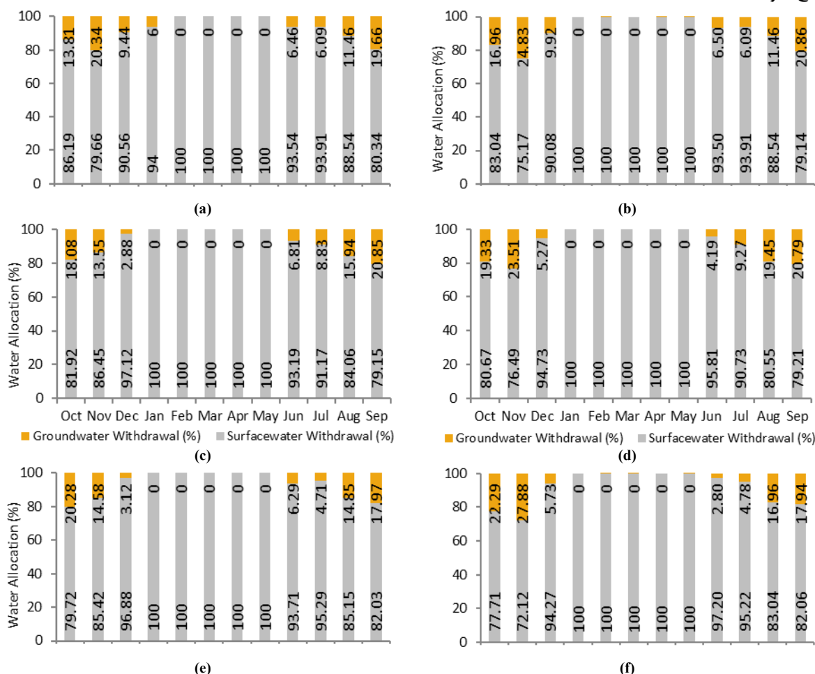
شکل ۱۰. درصد تخصیص از منابع آب سطحی و زیرزمینی: a و b: سناریوی اول و دوم در دز شرقی، c و d: سناریوی اول و دوم در دز غربی، e و f: سناریوی اول و دوم در اراضی شاوور
