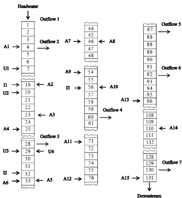
شکل ۳. بازه‌بندی رودخانه و منابع نقطه‌ای ورودی و خروجی
