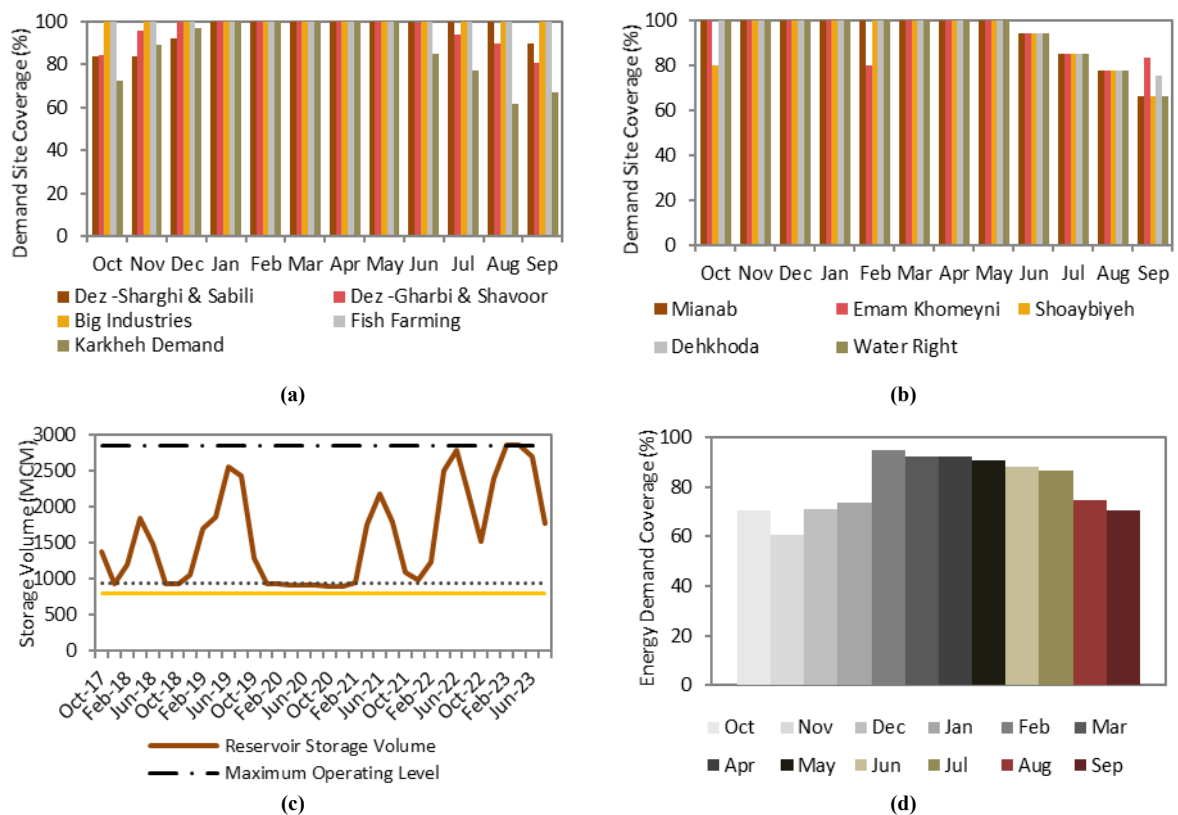
شکل ۶. نتایج اجرای سناریوی اول: a- متوسط درصد تأمین نیاز مصارف بالادست منطقه مطالعاتی دز b- متوسط درصد تأمین نیاز مصارف پایین دست منطقه مطالعاتی c- تغییرات حجم ذخیره ماهانه مخزن سد در طول دوره بهره‌برداری ۶ ساله d- متوسط درصد تأمین نیاز برق تولیدی
