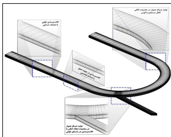
شکل ۸- شبکه‌بندی میدان حل با کلاستر بندی‌های مختلف در جهات متفاوت
