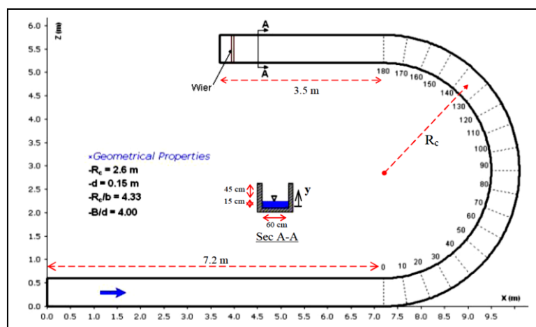
شکل ۲- مشخصات هندسی مدل آزمایشگاهی قوس ۱۸۰ درجه
