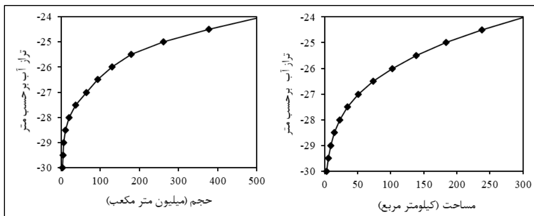
شکل ۳- منحنی سطح-حجم-ارتفاع تالاب انزلی (Modaberi and Shokoohi, 2019)
