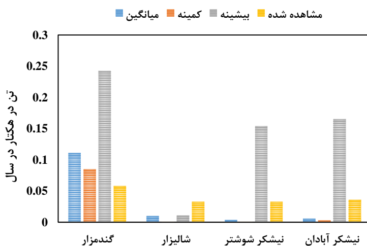
شکل ۶- مقایسه شار اکسید نیتریک در بین ایستگاه‌های مورد مطالعه
