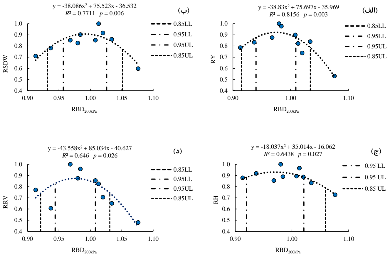
شکل ۲- روابط چگالی ظاهری نسبی بدست آمده از تنش محوری ۲۰۰ کیلو پاسکال در فشردگی محصور (RBD 200kPa ) با جرم محصول دانه نسبی (RY) (الف)؛ جرم خشک ساقه و برگ نسبی (RSDW) (ب)؛ ارتفاع گیاه نسبی (RH) (ج) و حجم ریشه نسبی (RRV) (د)
