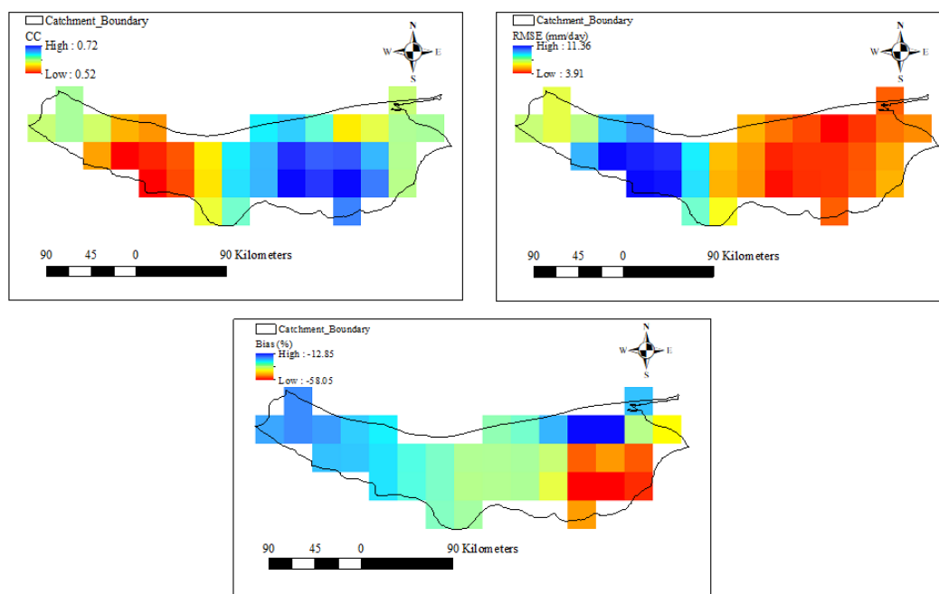
شکل ۶- تغییرات مکانی شاخص‌های CC، RMSE و Bias بارش شبیه‌سازی شده در سطح استان مازندران (مرحله واسنجی)
