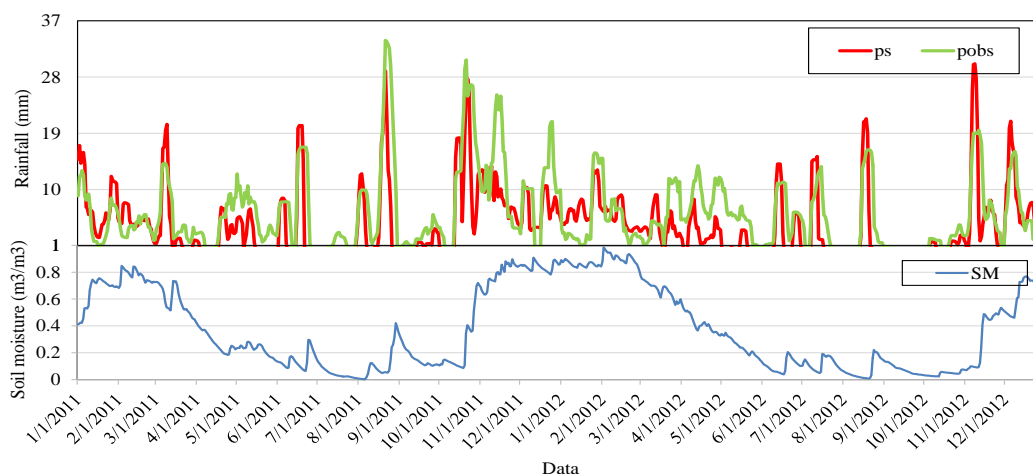
شکل ۹- صحت‌سنجی الگوریتم SM2RAIN در سطح استان مازندران در بازه زمانی ۲۰۱۱-۲۰۱۳ (Pobs: بارش مشاهداتی، Ps: بارش شبیه‌سازی شده)
