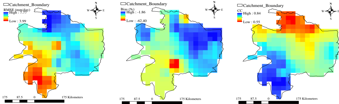
شکل ۲- تغییرات مکانی شاخص‌های RMSE، Bias و CC بارش شبیه‌سازی شده در سطح استان خراسان رضوی (مرحله واسنجی)
