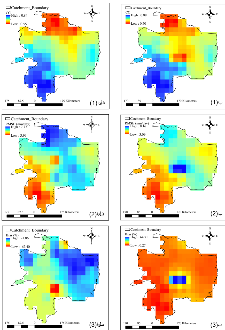
شکل ۱۰- نقشه توزیع مکانی شاخص‌های CC، RMSE و Bias بارش شبیه‌سازی شده توسط الگوریتم SM2RAIN در سطح استان خراسان رضوی (مرحله واسنجی) (گروه الف بدون لحاظ کردن تبخیر-تغرق و گروه ب بعد از اضافه کردن ترم تبخیر-تغرق به معادله بیلان آب خاک)
