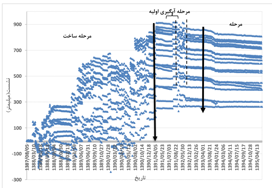
شکل ۳- نشست قائم سد ایوشان نسبت به زمان در سه مرحله ساخت، اولین آگیری و بهره‌برداری (ابزار IS229)
