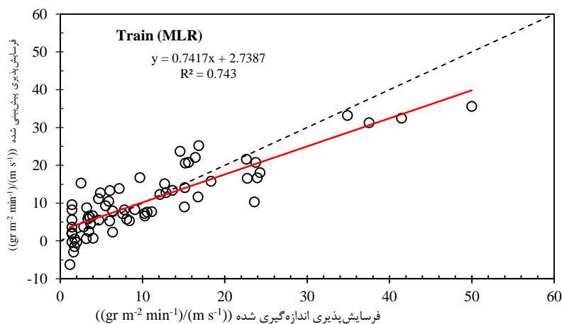
شکل ۸- مقایسه مقادیر فرسایش‌پذیری اندازه‌گیری شده در تونل باد و مقادیر فرسایش‌پذیری پیش‌بینی شده توسط مدل‌ها برای دو بخش آموزش و آزمون
