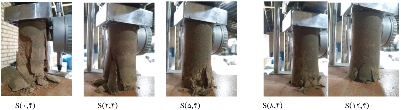
شکل ۱۰. تصویر نمونه‌های با ۴ درصد آهک و درصد‌های مختلف خاکستر باگاس پس از گسیختگی در زمان عمل آوری ۲۸ روزه
