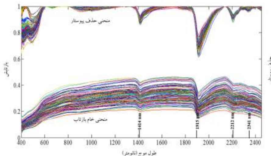
شکل ۵. میانگین منحنی‌های خام و حذف پیوستار بازتاب طیفی خاک‌های مورد مطالعه، موقعیت مشخصه‌های جذبی در طول موج‌های ۱۴۱۴، ۱۹۱۵، ۲۲۱۲ و ۲۳۴۱ نانومتر بر روی شکل مشخص شده است.
