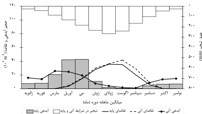
شکل ۳. میانگین ماهیانه حجم آبدهی به مخزن و میانگین ماهیانه عمق تبخیر همراه میانگین ماهیانه حجم تقاضای آب در شرایط پایه و تغییر اقلیم
