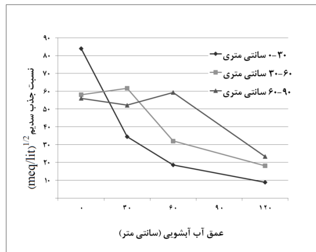
شکل ۵. روند تغییرات نسبت جذب سدیم عصاره اشباع خاک با آبخویی با آب کارون در اعماق مختلف
