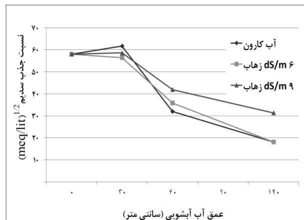
شکل ۳. روند تغییرات نسبت جذب سدیم عصاره اشباع خاک در عمق ۳۰ تا ۶۰ سانتی متری
