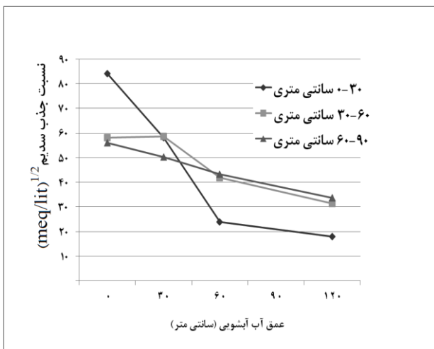
شکل ۷. روند تغییرات نسبت جذب سدیم عصاره اشباع خاک با آبخویی با زهاب با شوری ۹۱۰ dS/m در اعماق مختلف
