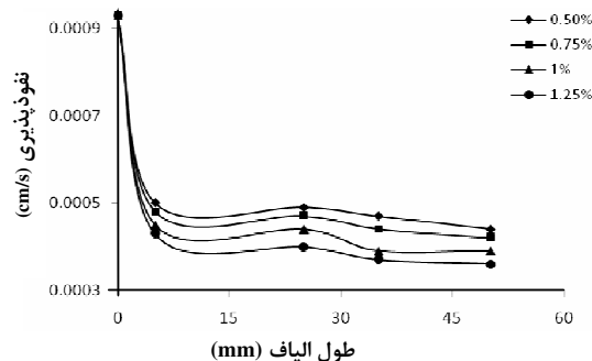
شکل ۴. تغییرات نفوذپذیری خاک با درصد‌های مختلف الیاف مصنوعی
