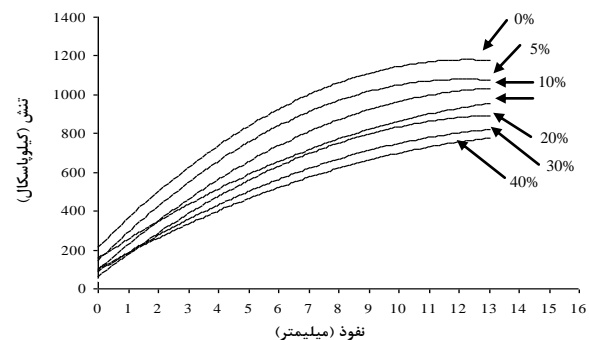
شکل 10- نتایج آزمایش CBR روی نمونه های مصنوعاً گچی شده (قبل از آبتشویی)
