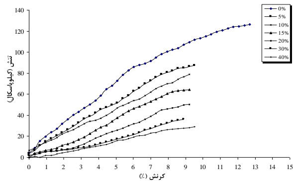
شکل 9- نتایج آزمایش تک محوری روی نمونه های مصنوعاً گچی شده (پس از آبتشویی)
