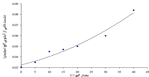
شکل 11- رابطه مقدار گچ و نشست ناشی از آبتشویی نمونه های مصنوعاً گچی شده
