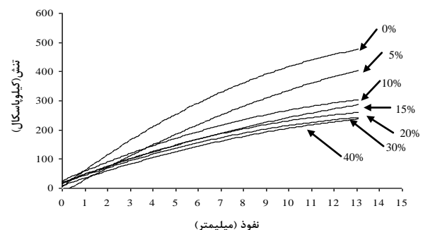
شکل 11- نتایج آزمایش CBR روی نمونه های مصنوعاً گچی شده (پس از آبتشویی)
