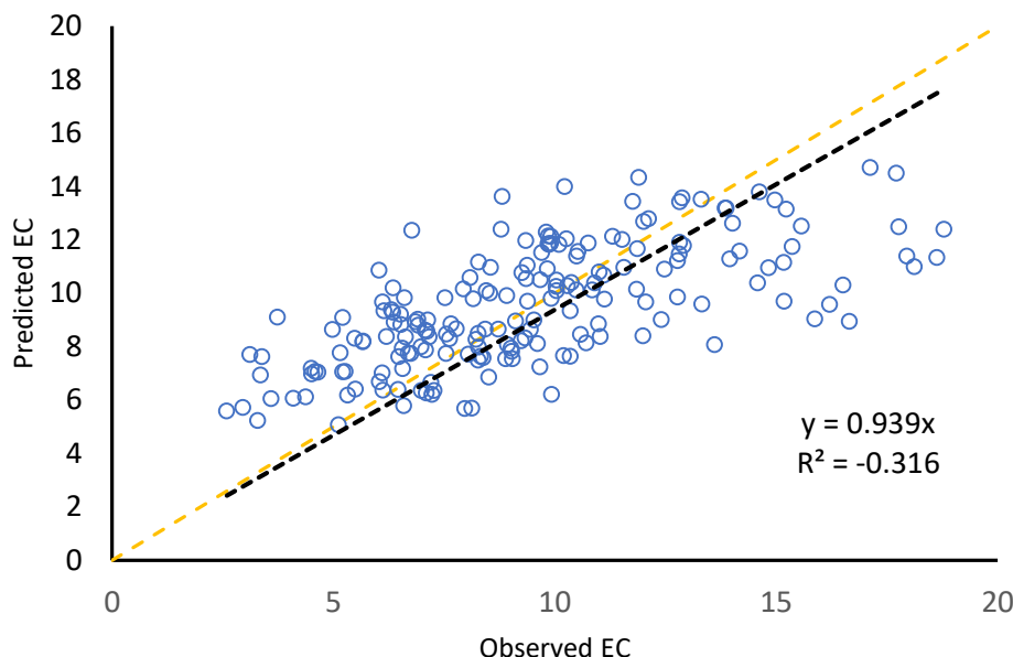
شکل ۴- همبستگی بین مقادیر اندازه‌گیری و پیش‌بینی شده توسط جنگل تصادفی در دسته آزمون
