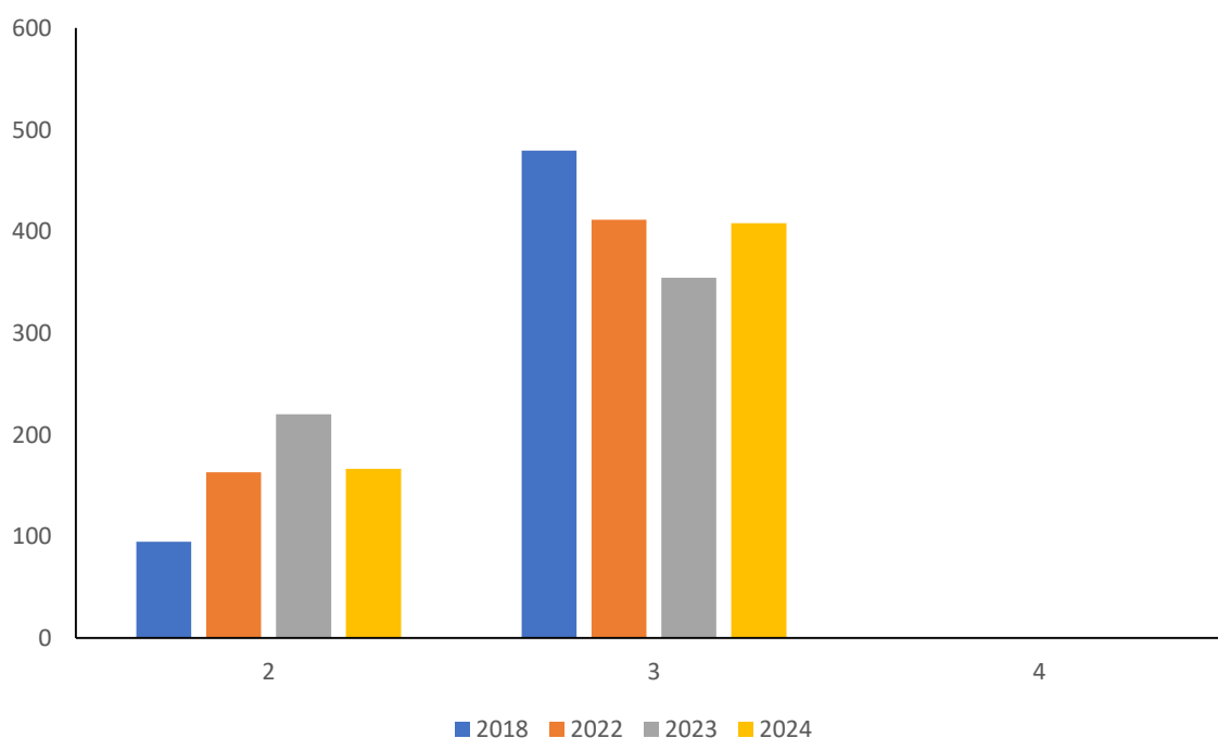
شکل ۵- نقشه و نمودار تغییرات میانگین شوری خاک پروژه زهکشی و بهسازی خاک تنور لاهور در استان یزد
