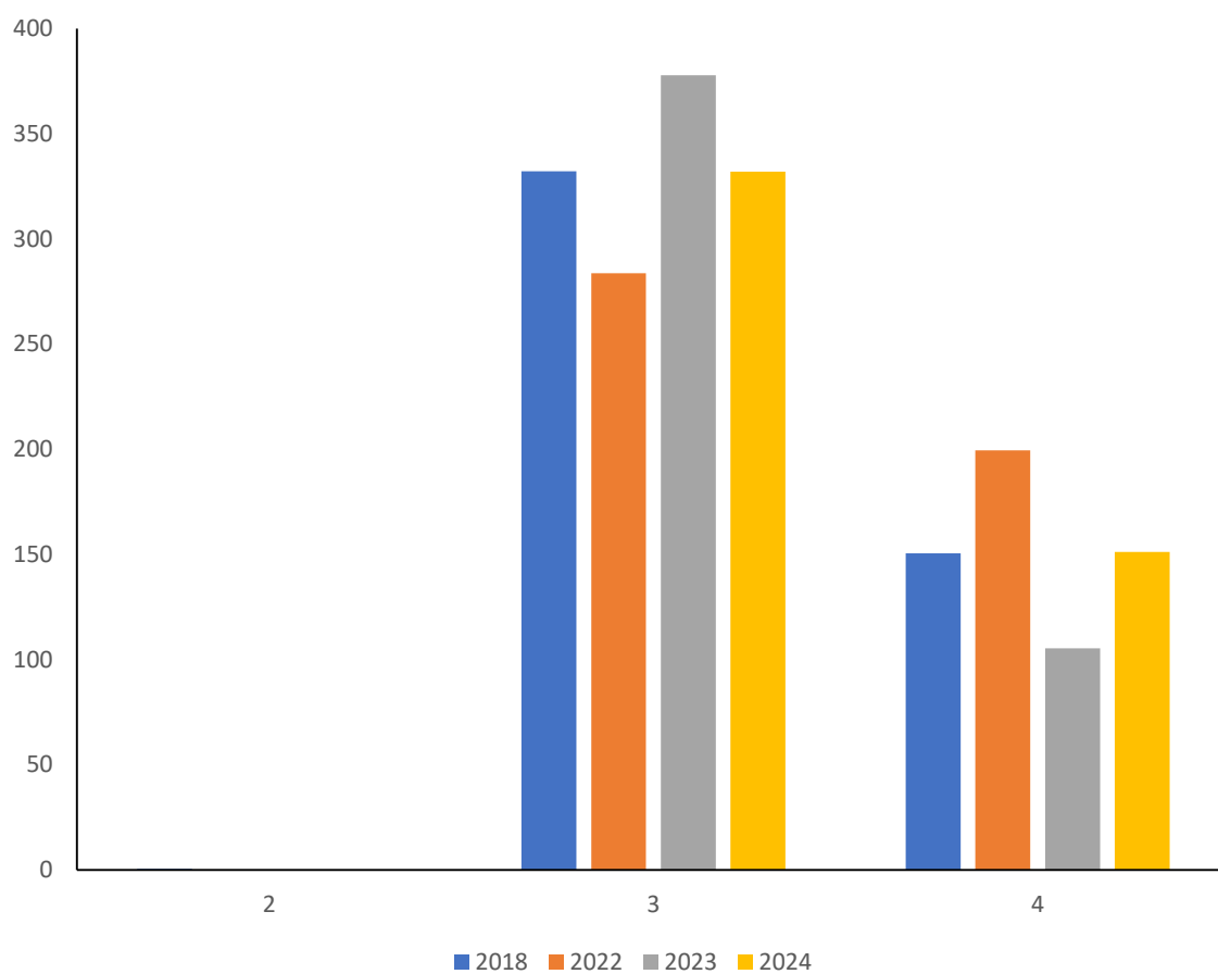
شکل ۶- نقشه و نمودار تغییرات میانگین شوری خاک باغ مرتاضیه در استان یزد
