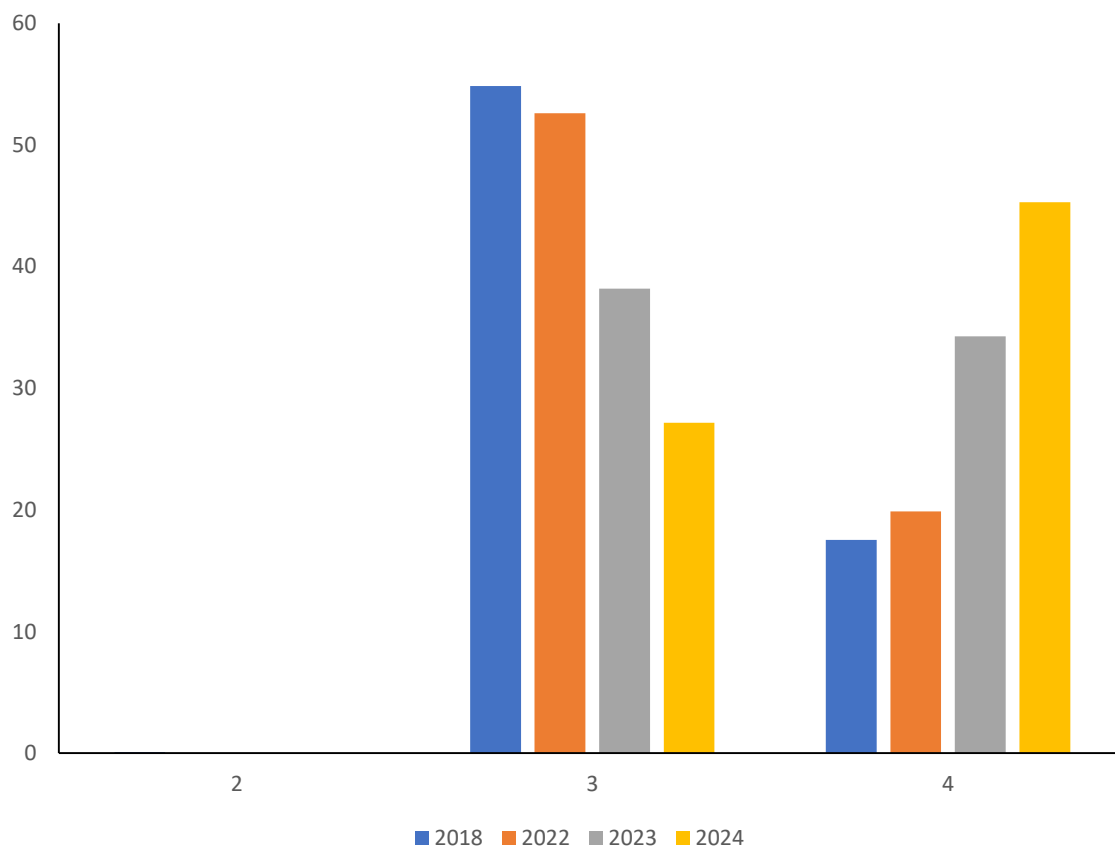
شکل ۷- نقشه و نمودار تغییرات میانگین شوری خاک باغ رضایی در استان یزد
