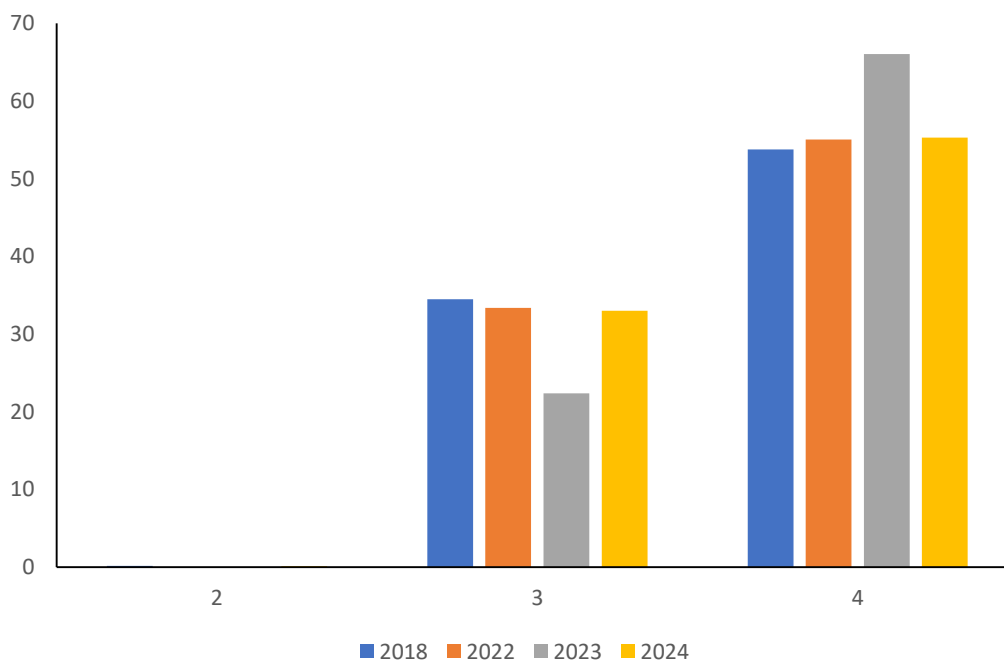
شکل ۸- نقشه و نمودار تغییرات میانگین شوری خاک باغ دادیار در استان خراسان رضوی
