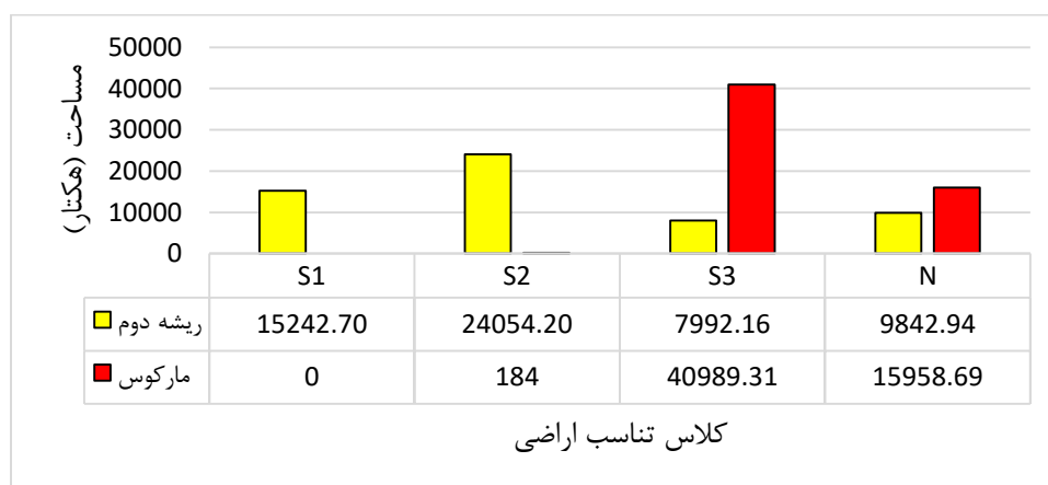
شکل ۵. مقایسه مساحت کلاس‌های تناسب اراضی در روش‌های مارکوس و ریشه دوم
