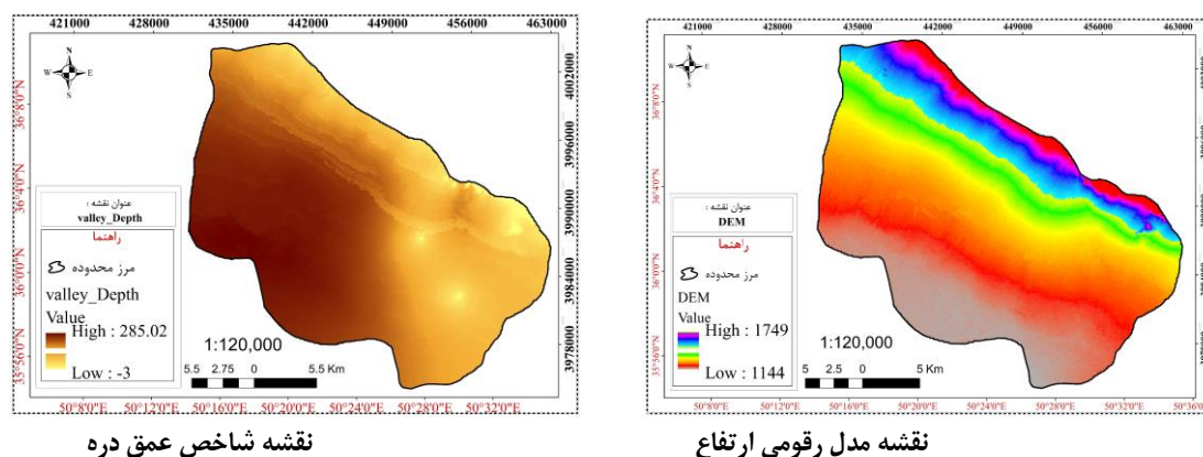
شکل ۴. نقشه متغیرهای محیطی استفاده شده در تهیه نقشه رقومی تناسب اراضی
