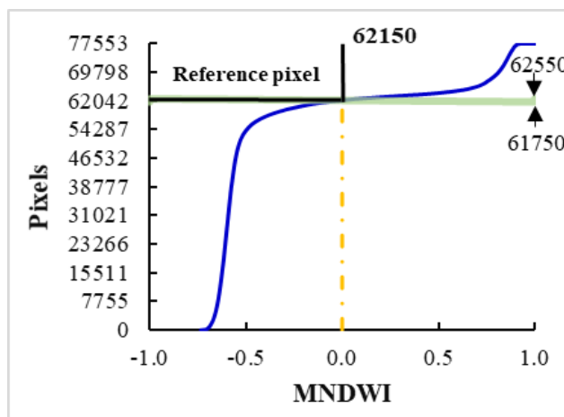
شکل ۷. نمودار فراوانی تجمعی داده‌ها و انتخاب پیکسل آستانه اولیه، ۱۱ فوریه ۲۰۱۶
