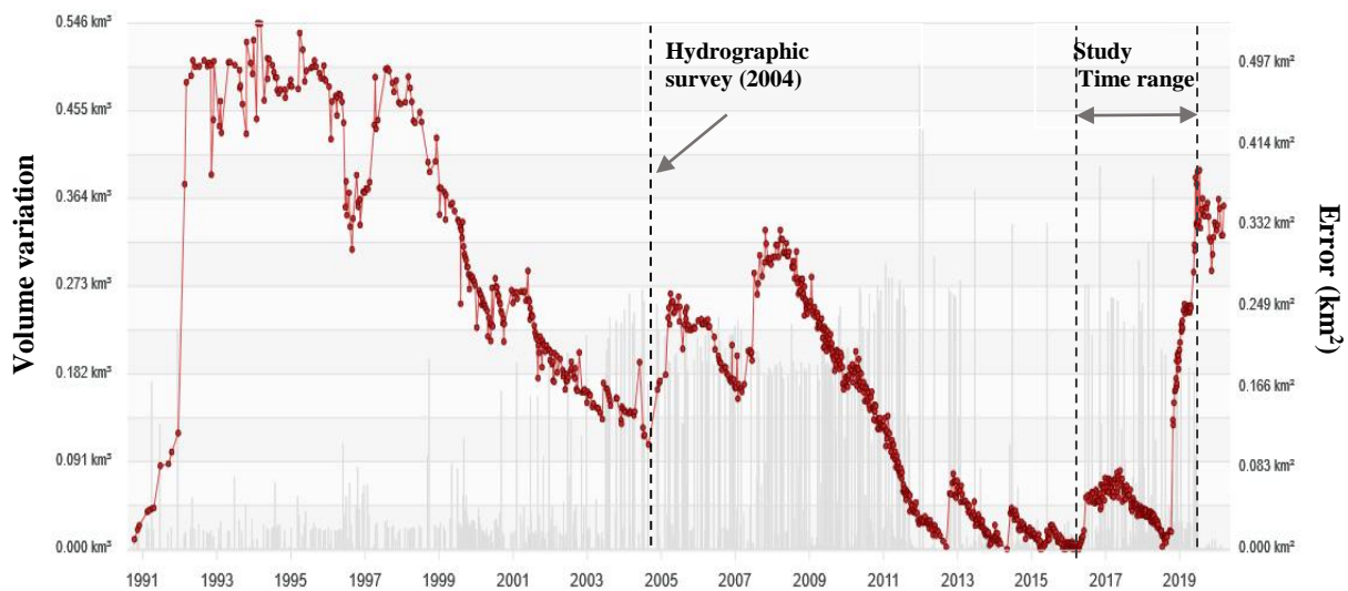
شکل ۴. داده‌های سری زمانی تغییرات حجم آب مخزن O. H. Ivie
