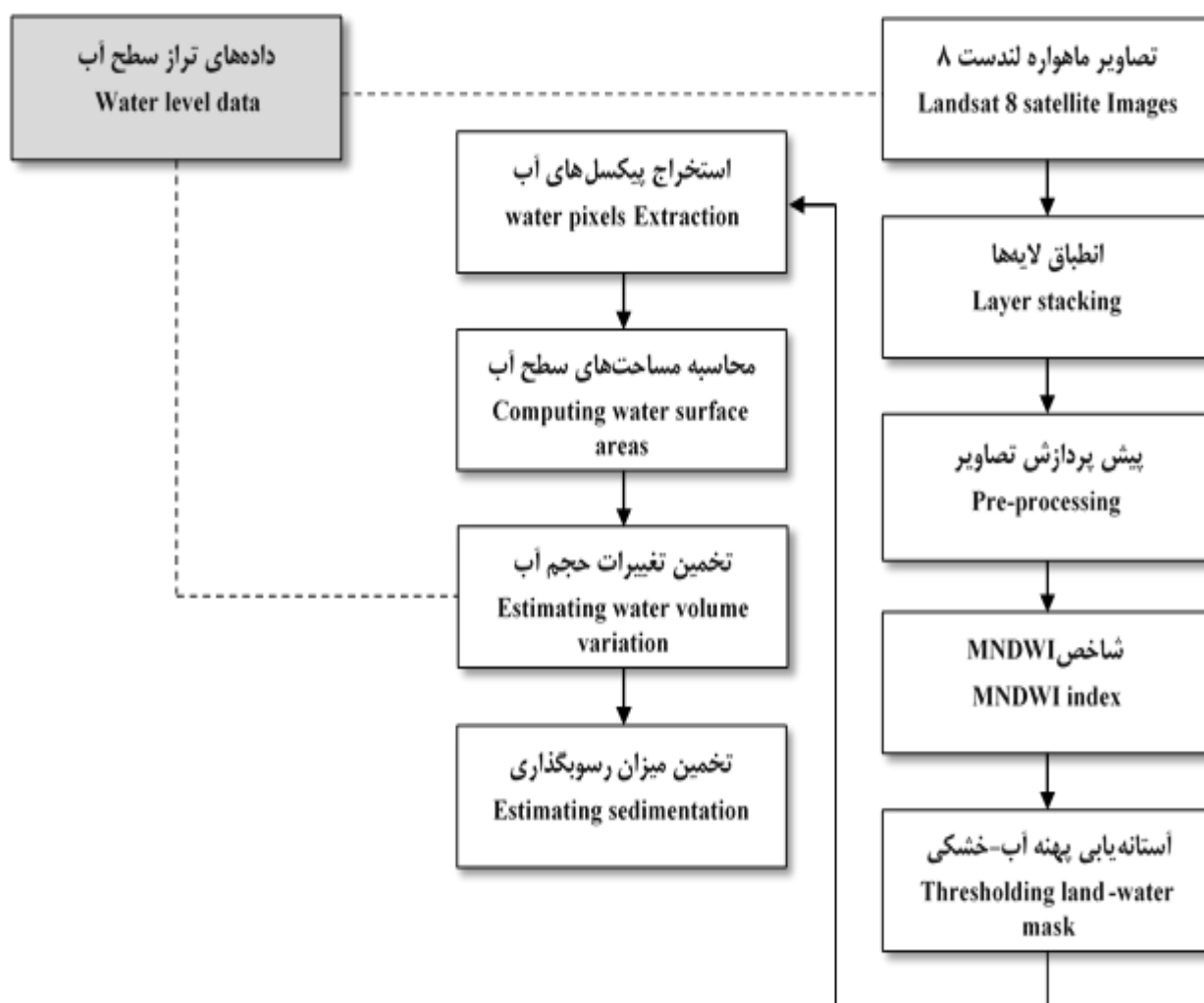
شکل ۱۰. فلوجارت تخمین میزان رسوب‌گذاری مخزن سد.
