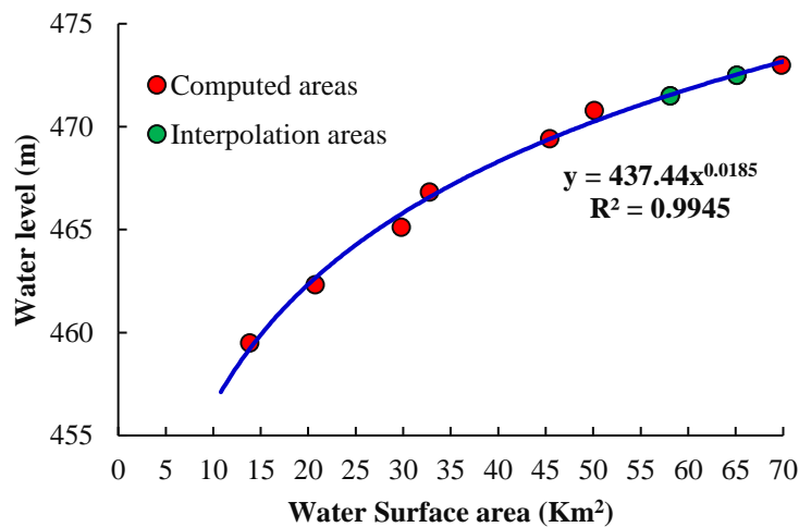
شکل ۹. منحنی ارتفاع-سطح مخزن O. H. Ivie با استفاده از مساحت‌های محاسبه شده بین سال‌های ۲۰۱۶ تا ۲۰۱۹.
