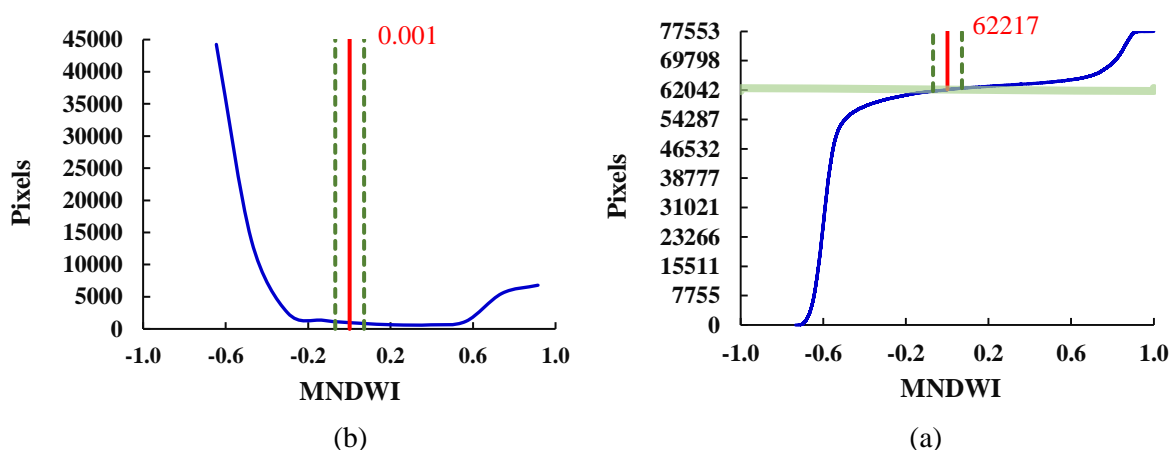
شکل ۸. پیکسل مرجع نهایی در نمودار تجمعی فراوانی (a) و آستانه مرجع نهایی در نمودار فراوانی (b)، ۱۱ فوریه ۲۰۱۶
