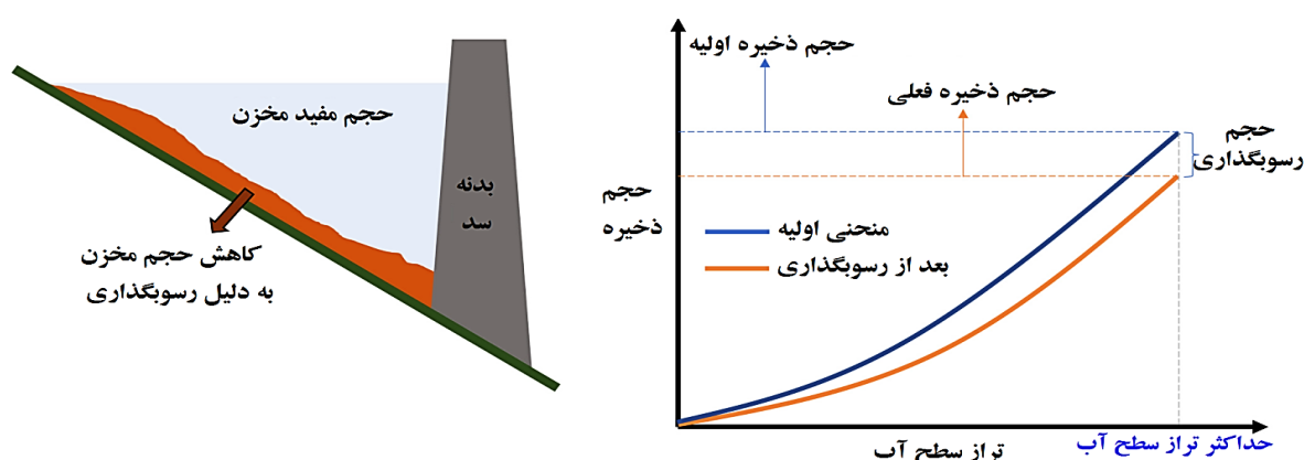
شکل ۱. نمای جانبی مخزن با رسوبات انباشته شده (a)، مقایسه منحنی ارتفاع-حجم اولیه مخزن با ترسیم شده بعد از گذشت زمان (b).
