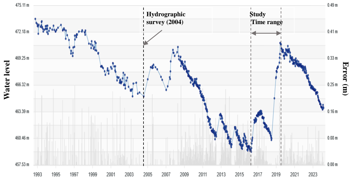
شکل ۳. داده‌های سری زمانی تراز سطح آب مخزن O. H. Ivie
