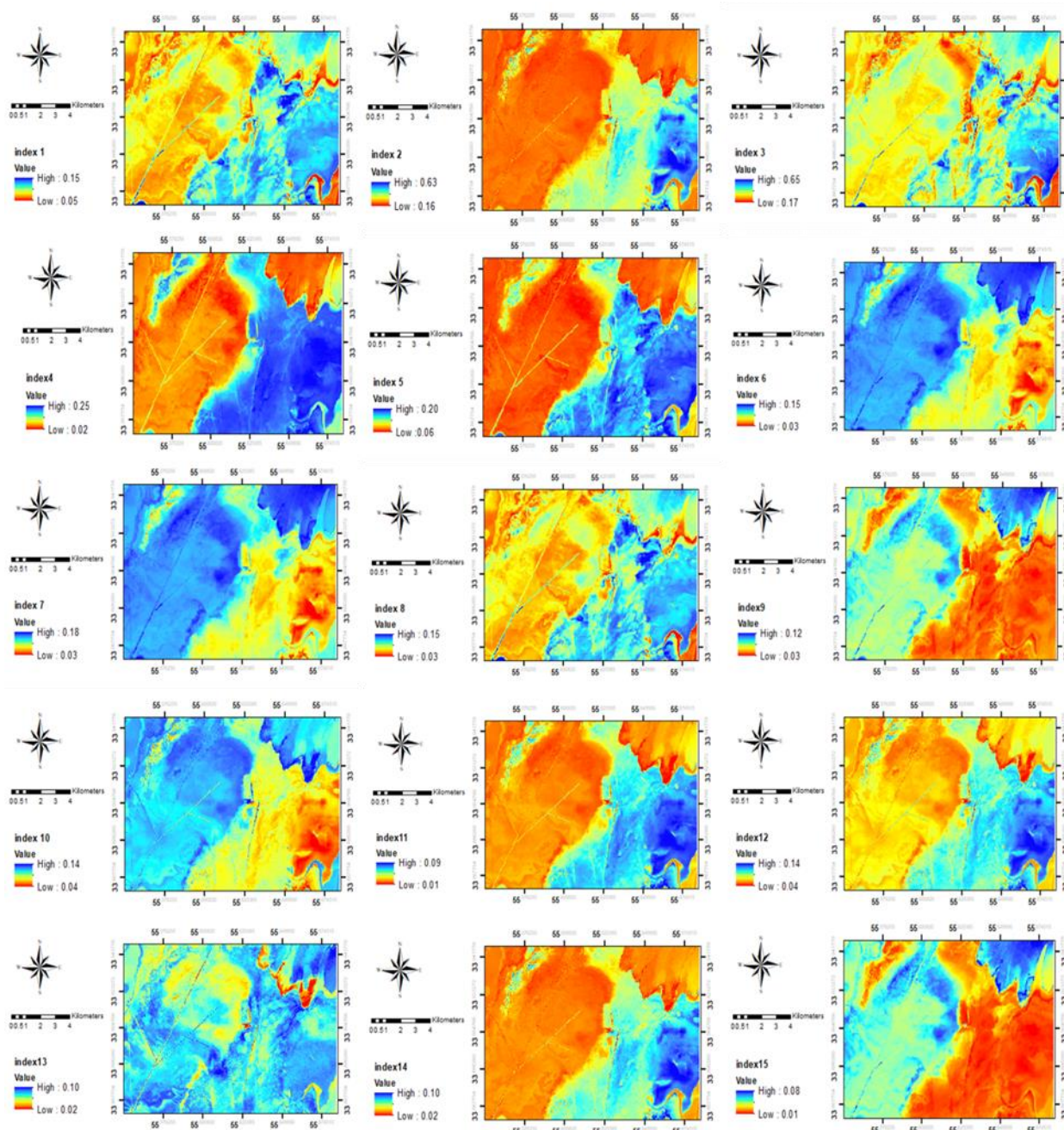
شکل ۳. نقشه ۱۵ شاخص ماهواره‌ای مورد استفاده در مطالعه بر اساس جدول ۱
