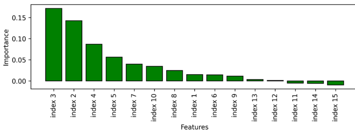
شکل ۷. نتایج بررسی اهمیت ویژگی‌ها و انتخاب آن‌ها بر اساس روش PFI برای مدل‌سازی مجدد با استفاده از الگوریتم RF
