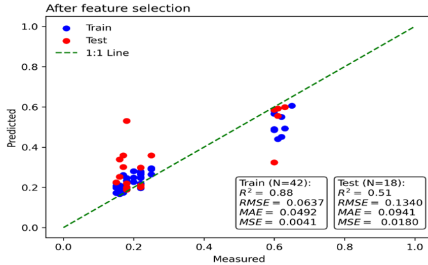
شکل ۸. نتایج واسنجی و صحت‌سنجی الگوریتم RF با استفاده از ۴ شاخص انتخاب شده بر اساس روش PFI
