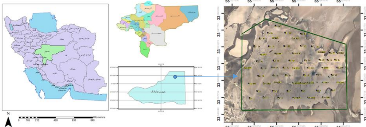
شکل ۱. موقعیت جغرافیایی منطقه مورد مطالعه و نمونه‌برداری شده در نقشه ایران و استان اصفهان، منطقه خور و بیابانک نمونه‌برداری، آماده‌سازی و اندازه‌گیری پتاسیم سطحی و عیار پتاسیم شورا به زیرزمینی
