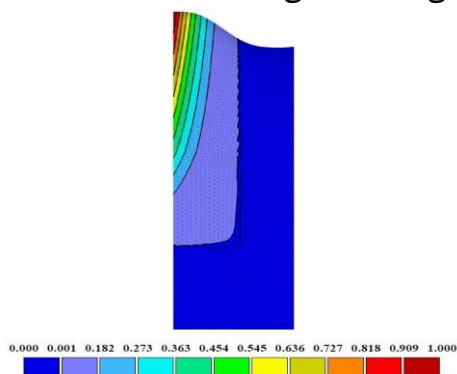
شکل ۲- توزیع ریشه ذرت و مقدار جذب آب از خاک در مدل HYDRUS-2D
