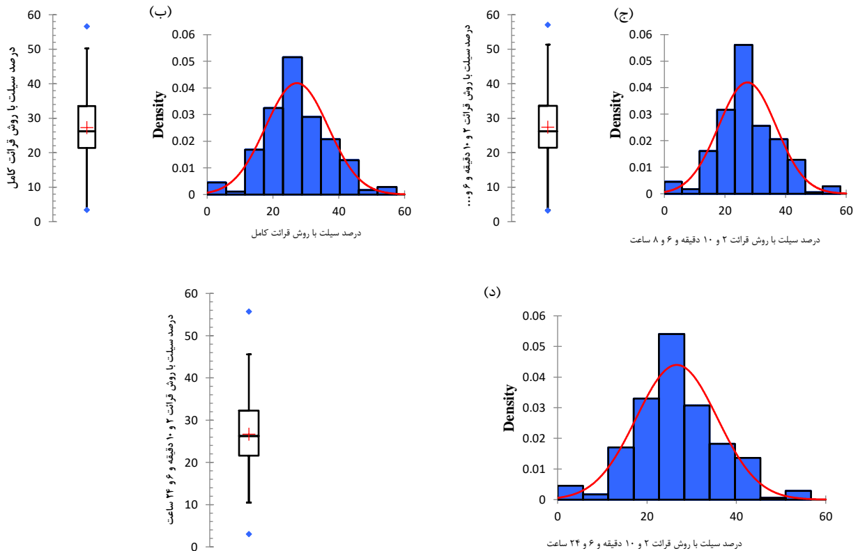
شکل ۱۲- مقایسه میانگین، نمودار جعبه‌ای (الف) و هیستوگرام همراه با برازش منحنی چگالی برای بخش سیلت اندازه‌گیری شده با روش‌های مختلف (ب- (در نمودار جعبه‌ای میانگین، میانه، ماکزیمم و مینیمم مؤثر و واقعی مشخص شده است). گروه‌های دارای حروف مشابه (a و b) در یک گروه قرار گرفته و از لحاظ آماری تفاوت معنی‌داری با یکدیگر ندارند.
