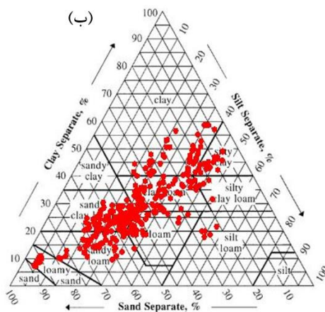
شکل ۸- کلاس بافتی تعیین شده منتج از روش چهار قرائت ۲ و ۱۰ دقیقه و ۲۴ ساعت و مقایسه آن با روش قرائت کامل بر مبنای طبقه‌بندی انجمن بین‌المللی علوم خاک (ISSS)
