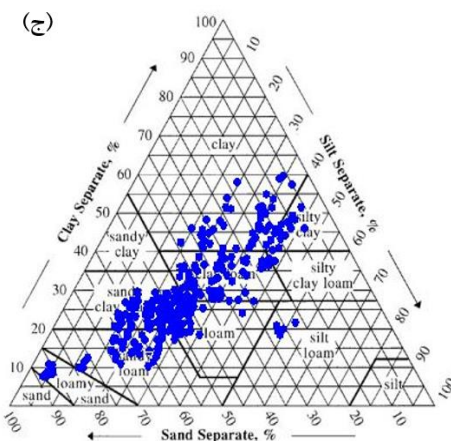
شکل ۸- کلاس بافتی تعیین شده منتج از روش چهار قرائت ۲ و ۱۰ دقیقه و ۲۴ ساعت و مقایسه آن با روش قرائت کامل بر مبنای طبقه‌بندی انجمن بین‌المللی علوم خاک (ISSS)
