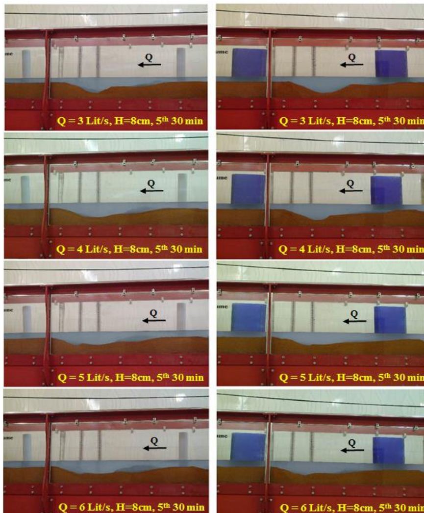
شکل ۱۲. تأثیر دبی بر روی آبستگی ایجاد شده در اطراف پایه‌های پل در اثر توسعه گودال برداشت مصالح
