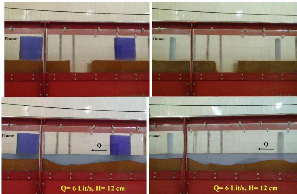
شکل ۸. انتقال حفره برداشت مصالح به پایه‌های پل مستقر در بالادست و پایین دست
