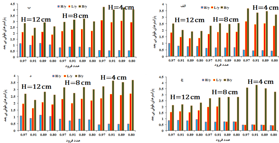
شکل ۱۶. تغییرات پارامترهای بی‌بعد H/y ، L/y و B/y برای حداکثر عمق آبستتگی (الف) پایه پل دایره‌ای شکل (۰/۱۵ میلی‌متری)، (ب) پایه پل دایره‌ای شکل (۰/۰۶ میلی‌متری) (ج) پایه پل مستطیلی نوک تیز (۰/۱۵ میلی‌متری)، (د) پایه پل مستطیلی نوک تیز (۰/۰۶ میلی‌متری)
