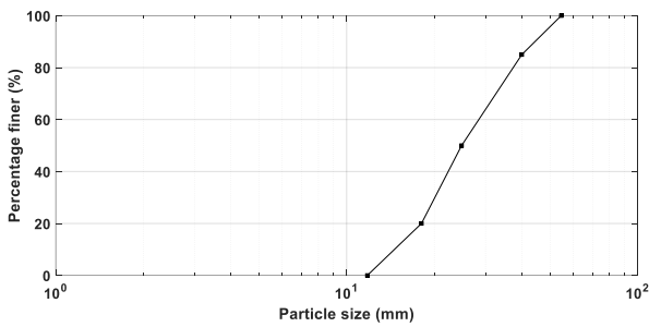
شکل ۴- منحنی دانه بندی ذرات گرد گوشه
