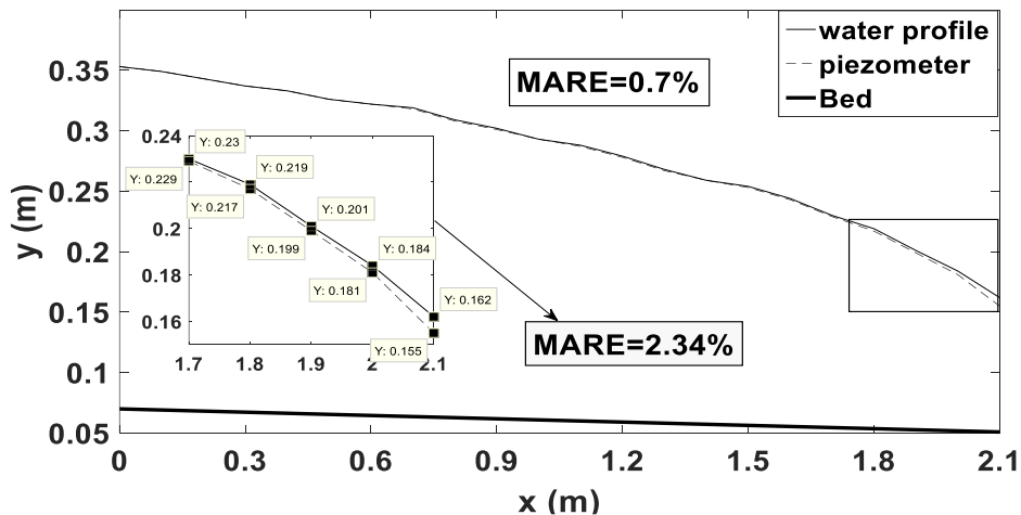
شکل ۶- مقادیر آزمایشگاهی نیمرخ طولی سطح آب و نیمرخ فشار وارد بر کف برای دبی ۱/۲۷ لیتر بر ثانیه و مصالح گردگوشه با قطر متوسط ۲۶ میلی‌متر
