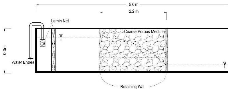
شکل ۲- نمای نیمرخ طولی مدل آزمایشگاهی
