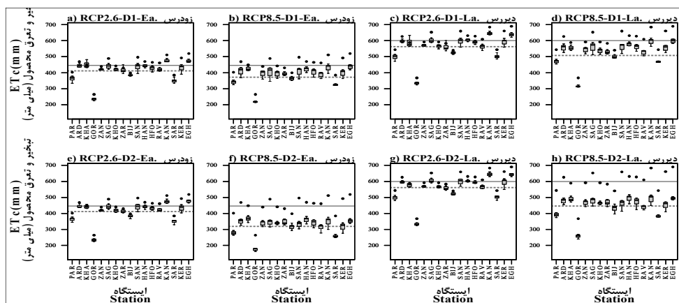
شکل ۳- متوسط مجموع تبخیر و تعرق محصول ( E_{Tc} ) طی دوره رشد برای دوره پایه (دایره‌های توپر) ۲۰۰۵-۱۹۷۵ و پیش‌نگری‌های اقلیمی هفت مدل GCM (نمودار جعبه‌ای) برای هر ایستگاه. a, b, c و d مربوط به دوره D1 (۲۰۴۵-۲۰۶۵) و سناریوهای RCP2.6 و RCP8.5 و ارقام زودرس (Ea.) و دیررس (La.). به همین ترتیب برای e, f, g و h اما برای دوره D2 (۲۰۸۰-۲۱۰۰). متوسط مجموع تبخیر و تعرق محصول ( E_{Tc} ) طی دوره رشد برای تمام ایستگاه‌ها در دوره پایه و آینده به ترتیب با خطوط ممتد و منقطع در هر نمودار نشان داده شده است. ایستگاه‌ها بر روی محور افقی از شمال به جنوب مرتب شده است.
