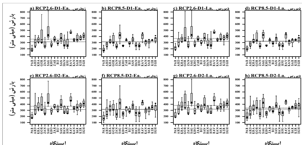
شکل ۲- متوسط مجموع بارش طی دوره رشد برای دوره پایه (دایره‌های توپر) ۲۰۰۵-۱۹۷۵ و پیش‌نگری‌های اقلیمی هفت مدل GCM (نمودار جعبه‌ای) برای هر ایستگاه. a, b, c و d مربوط به دوره D1 (۲۰۴۵-۲۰۶۵) و سناریوهای RCP2.6 و RCP8.5 و ارقام زودرس (Ea.) و دیررس (La.). به همین ترتیب برای e, f, g و h اما برای دوره D2 (۲۰۸۰-۲۱۰۰). متوسط مجموع بارش طی دوره رشد برای تمام ایستگاه‌ها در دوره پایه و آینده به ترتیب با خطوط ممتد و منقطع در هر نمودار نشان داده شده است. ایستگاه‌ها بر روی محور افقی از شمال به جنوب مرتب شده است.
