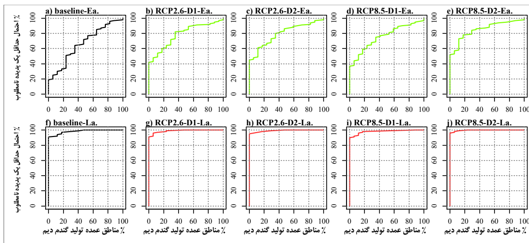
شکل ۵- احتمال تجمعی وقوع حداقل یک پدیده نامطلوب طی دوره رشد در برابر مناطق عمده تولید گندم دیم، (a) تا (e) برای رقم زودرس و (f) تا (j) برای رقم دیررس. برای دوره پایه (baseline) و متوسط پیش‌نگری‌های هفت مدل انتخابی GCM تحت سناریوهای RCP2.6 و RCP8.5 در دوره D1 (۲۰۴۵-۲۰۶۵) و دوره D2 (۲۰۸۰-۲۱۰۰).
