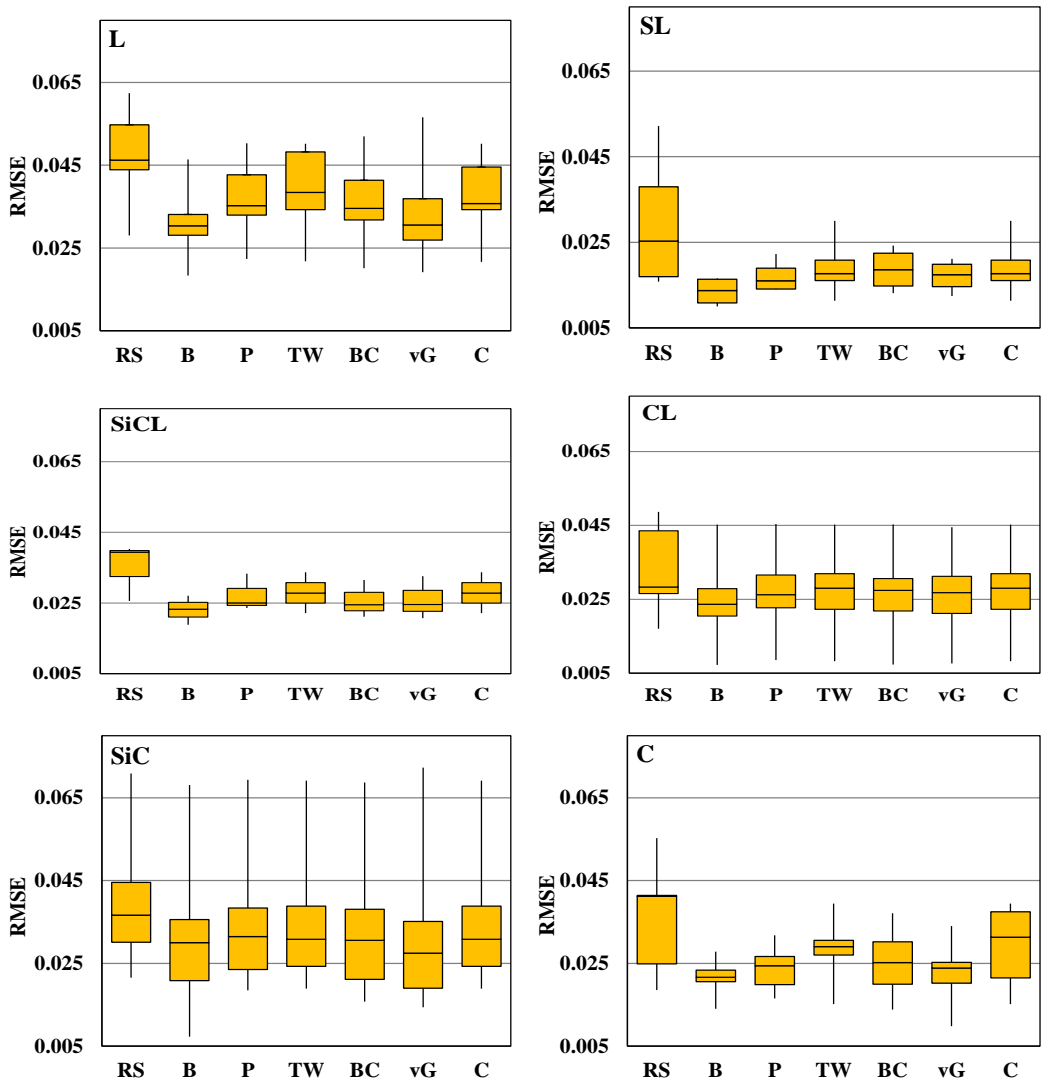
شکل ۶- نمودارهای جعبه‌ای ریشه میانگین مربعات خطا (RMSE) مربوط به مدل‌های فرکتالی منحنی مشخصه رطوبتی شامل Brooks (RS) و Rieu and Sposito (1991) (B)، Bird et al. (2000) (P)، Perfect (1999) (TW) و Tyler and Wheatcraft (1990) (TW) و مدل‌های تجربی شامل Brooks (RS) و Rieu and Sposito (1991) (B)، Bird et al. (2000) (B)، Perfect (1999) (P)، Tyler and Wheatcraft (1990) (TW) و Van Genuchten (1980) (vG) and Corey (1964) (BC)، برای کلاس‌های بافتی رس (C)، رس سیلتی (SiC)، لوم رس سیلتی (SiCL)، لوم رسی (CL)، لوم شنی (SL) و لوم (L)
