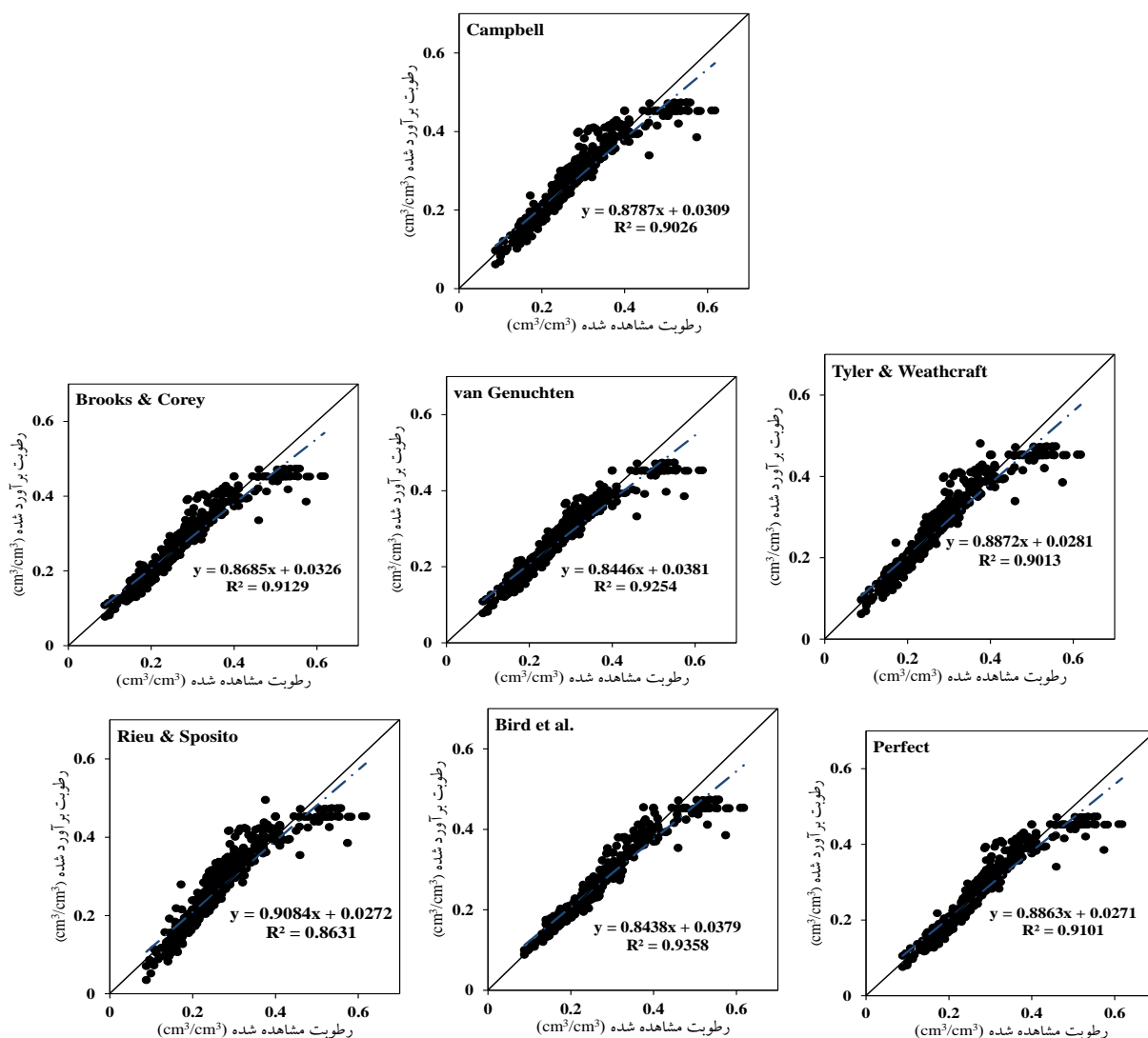
شکل ۴- مقادیر رطوبتی اندازه‌گیری شده در برابر مقادیر برآورد شده آن‌ها توسط مدل‌های فرکتالی (Rieu and Sposito (1991)، Bird et al. (2000)، Perfect (1999) و Tyler and Wheatcraft (1990) و مدل‌های تجربی (Brooks and Corey (1964) و Van Genuchten (1980) و Campbell (1974)). خط پیوسته قطری بیان‌گر خط ۱:۱ است.
