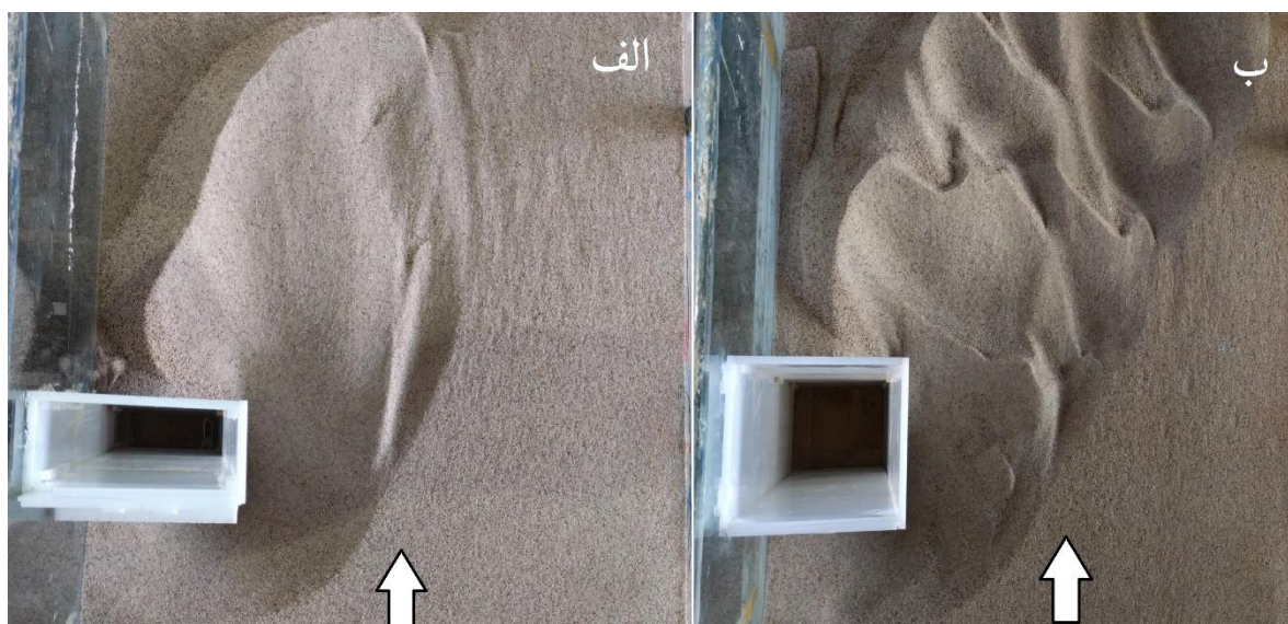
شکل ۱۱- وضعیت بستر پیرامون تکیه‌گاه در پایان آزمایش و در حالت بهینه: الف) تکیه‌گاه ۱ ب) تکیه‌گاه ۲
