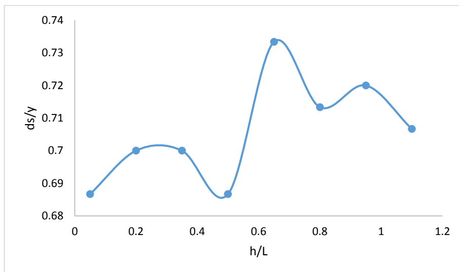
شکل ۵- تاثیر کارگذاری المان‌ها با اندازه ۰/۰۵L بالای سطح رسوب
