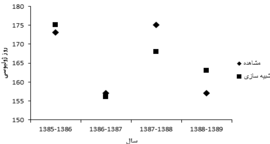
شکل ۲- تاریخ‌های رسیدن فنولوژیکی شبیه‌سازی شده و مشاهده‌ای گندم
