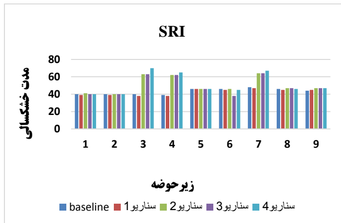
شکل ۷. الف-تداوم بر اساس شاخص SSWI. ب-تداوم بر اساس شاخص SRI
