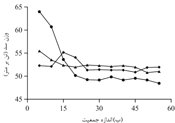
شکل ۷. تأثیر تعداد تکرار و اندازه جمعیت بر وزن سد برای ضرایب لغزش ۱/۵ و مقادیر مختلف ضریب لغزش
