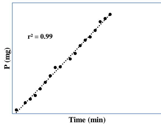
نمودار ۱. مقدار فسفر اندازه‌گیری شده در قسمت B از ابزار استفاده شده ( شکل ۳) در مقابل زمان
