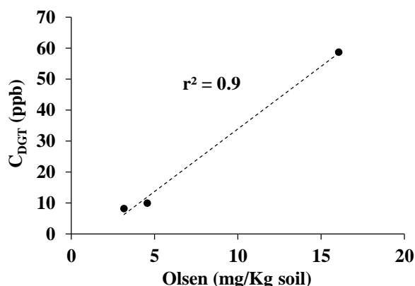
نمودار ۹. رابطه میزان فسفر اندازه‌گیری‌شده توسط DGT و روش اولسن
