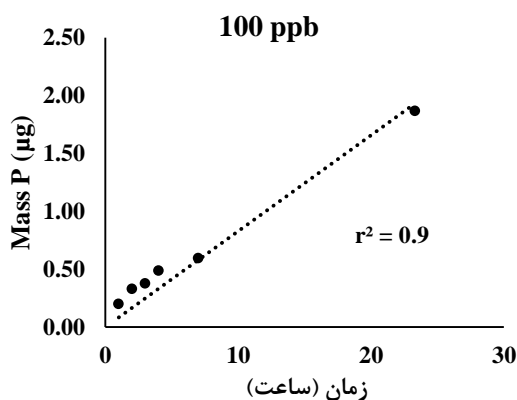
نمودار ۵. فسفر تجمع‌یافته در لایه جاذب DGT نسبت به زمان کاربرد در دو محلول با غلظت فسفر ۲۰۰ و ۱۰۰ ppb
