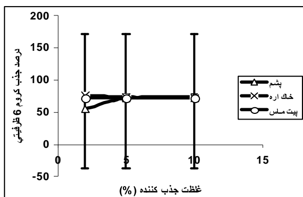
شکل ۱- اثر غلظتهای مختلف جذب کننده ها بر جذب کروم ۶ ظرفیتی در زمان ۲ روز در خاک خطوط نشان Standard Deviation است.
