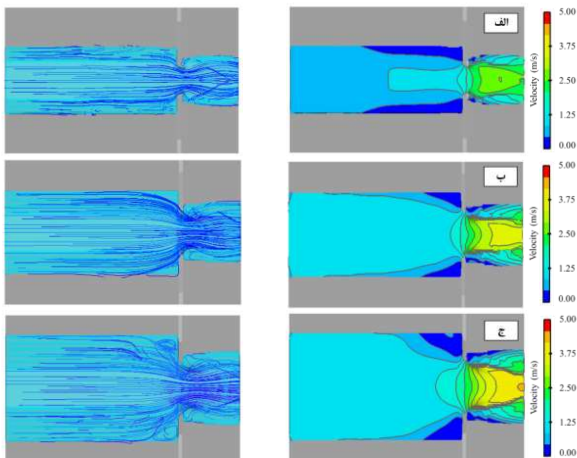
شکل ۱۱. میدان توزیع سرعت و خطوط جریان در دامنه محاسباتی شبیه‌سازی به‌ازاء دبی‌های الف) ۱، ب) ۲/۵ و ج) ۵ متر مکعب بر ثانیه
