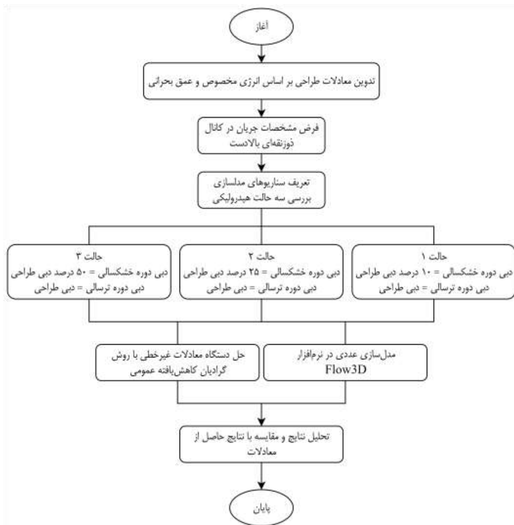
شکل ۳. روندنمای طراحی بررسی عملکرد شکاف کنترل مرکب دوونقه‌ای در شرایط مختلف هیدرولیکی
