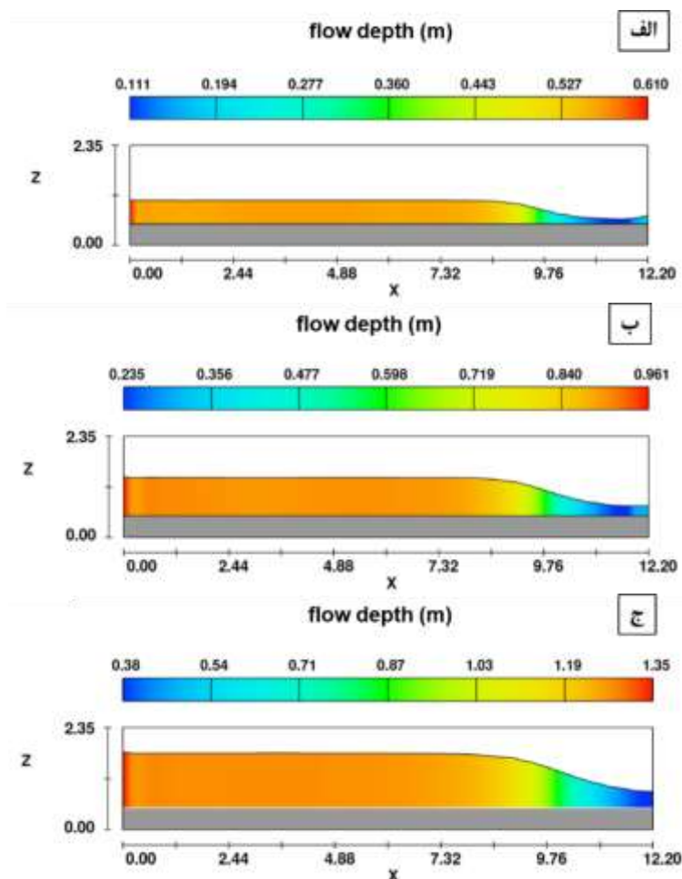
شکل ۹. نیمرخ سطح آب در حضور شکاف کنترل مرکب دوزنقه‌ای برای حالت‌های الف (۱، ۲ و ج) ۳
