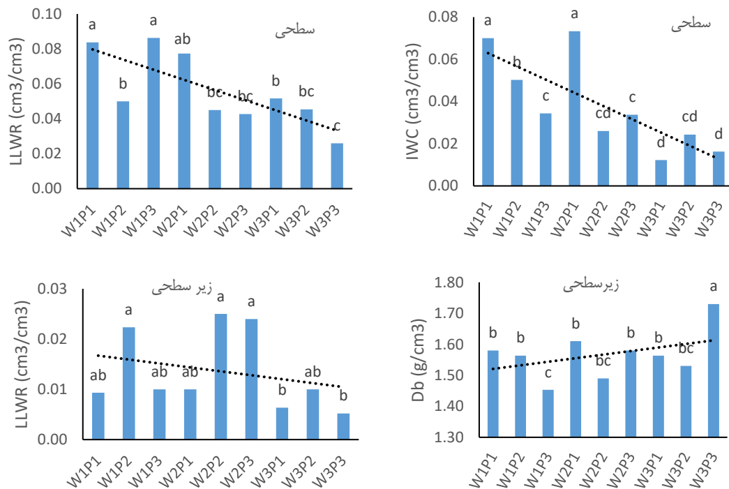
شکل ۲. مقایسه میانگین شاخص‌های LLWR و PAW و Db در لایه‌های سطحی و زیرسطحی
