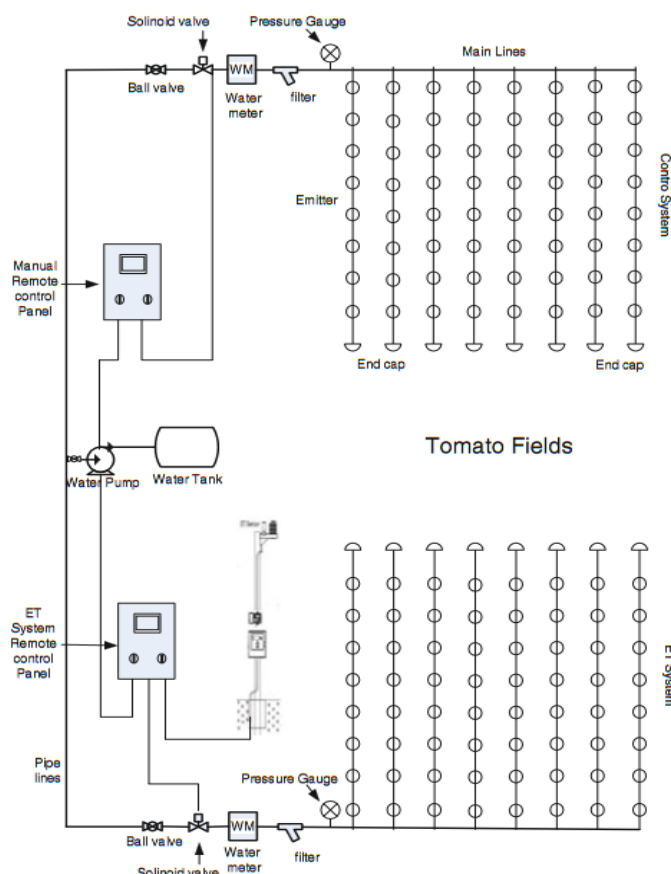
شکل ۹- نمونه یک سامانه آبیاری سنتی و هوشمند برای مزرعه گوجه‌فرنگی (Al-Ghobari & Mohammad, 2011)
