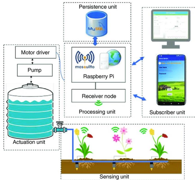
شکل ۱۹- شماتیکی از اجزای یک سامانه آبیاری کاملاً هوشمند مبتنی بر اینترنت اشیا (Dagar et al., 2018)
