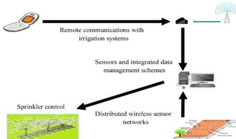
شکل ۱۵- رابطه فناوری مدیریت آبیاری با سنسور مستقل (Zhu et al., 2018)
