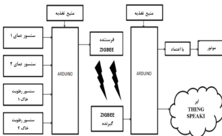
شکل ۱۳- سازمان‌دهی یک سامانه آبیاری هوشمند (Bagaria, 2019)
