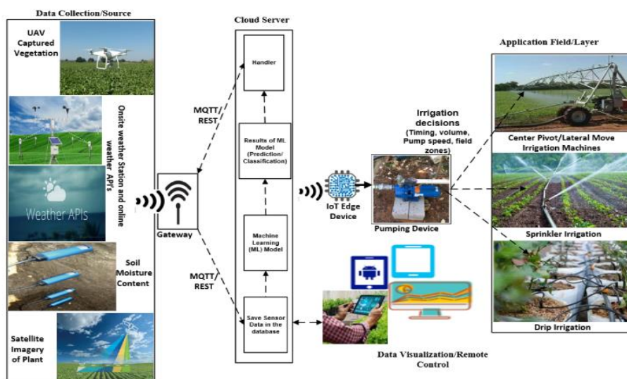
شکل ۱۶- لایه‌های معماری آبیاری مبتنی بر یادگیری ماشین با یک راه‌حل کشاورزی دیجیتال (Ayaz et al., 2019)
