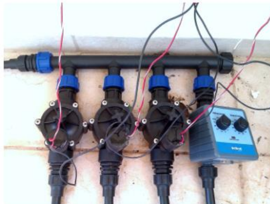
شکل ۴- نمایی از شیرهای سلنوییدی (Angelopoulos et al., 2011)
