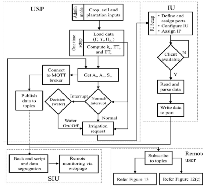
شکل ۱۴- جریان کار سامانه آبیاری هوشمند کم‌هزینه مبتنی بر شبکه عصبی (Nawandar & Satpute, 2019)
