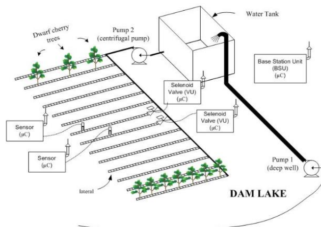
شکل ۵- نمای کلی از سامانه هوشمند آبیاری طراحی شده برای درختان گیلاس (Dursun & Ozden, 2011)
