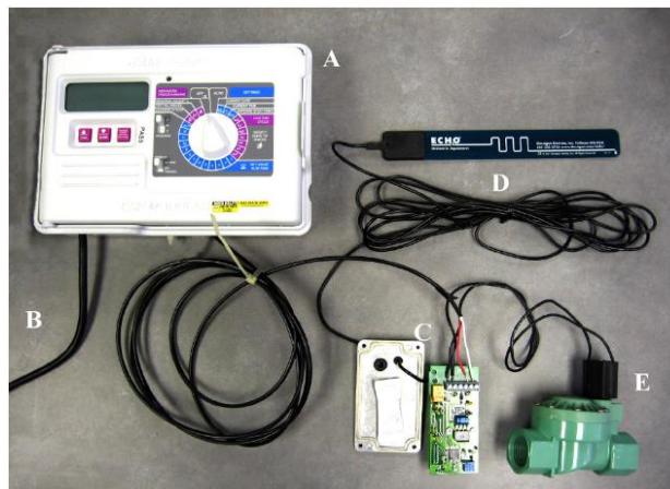
شکل ۱- نمایی از تجهیزات سامانه نیمه خودکار آبیاری برای گوجه فرنگی (Muñoz-Carpena & Dukes, 2005) A: سخت افزار کنترل زمان، B: منبع تغذیه، C: سنسور رطوبت سنج، D: پردازشگر زمان، E: شیر سلونوئیدی
