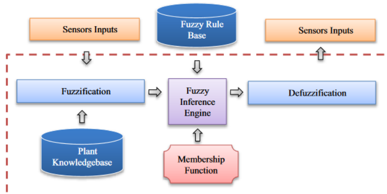
شکل ۱۱- کنترل‌کننده منطق فازی برای سامانه آبیاری هوشمند (Izzuddin et al., 2018)
