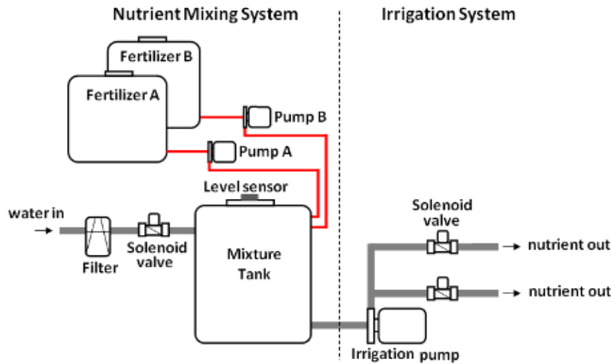
شکل ۷- نحوه عملکرد سامانه آبیاری توأم با کوددهی به صورت خودکار (Salih et al., 2011)
