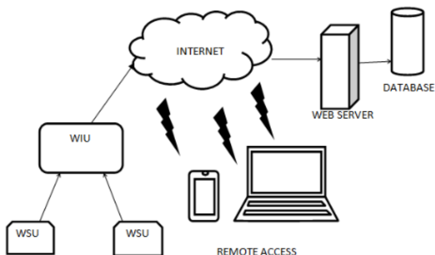
شکل ۱۲- مدل معماری سامانه پیشنهادی آبیاری هوشمند (Bagaria, 2019)
