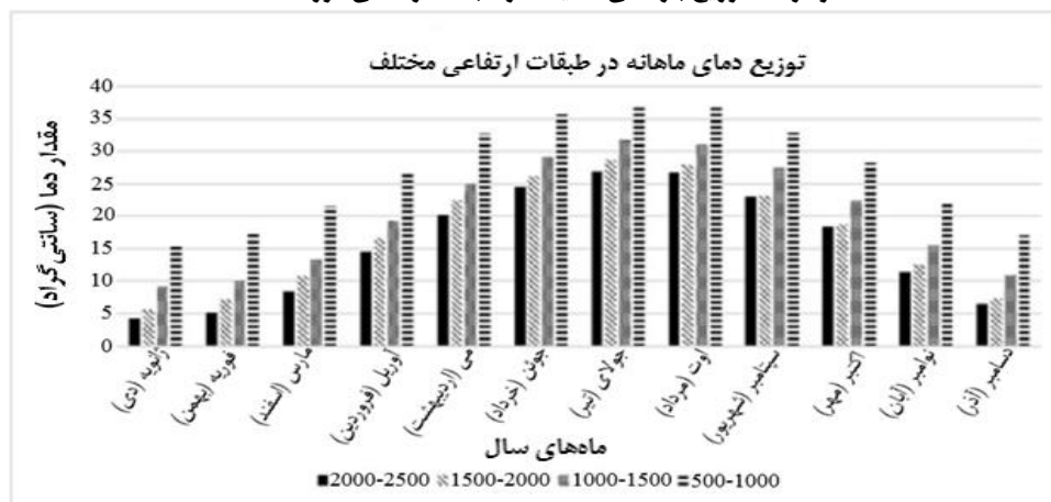
نمودار ۲- توزیع دما ماهیانه در طبقات ارتفاعی مورد مطالعه.
