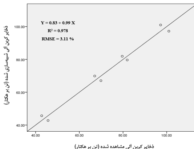
شکل ۴- اعتبارسنجی مدل با مقایسه داده‌های شبیه‌سازی شده و مشاهده شده ذخایر کربن آلی در هر چهار طبقه ارتفاعی در سال ۲۰۲۲
