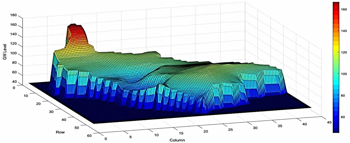
شکل ۱۲- نقشه سه بعدی تراز آب زیرزمینی دشت لور در پایان دوره شبیه سازی (سپتامبر ۲۰۵۰) در سناریوی SSP4-8.5 - بهترین مدل (MIROC)
