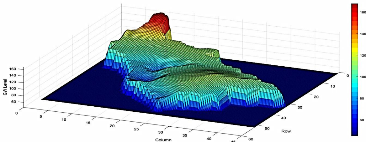
شکل ۱۱- نقشه سه‌بعدی تراز آب زیرزمینی دشت لور در پایان دوره شبیه‌سازی (سپتامبر ۲۰۵۰) در سناریوی SSP1-2.6 - بهترین مدل (MIROC)
