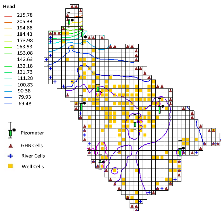
شکل ۴- واسنجی مدل آب زیرزمینی در حالت ماندگار
