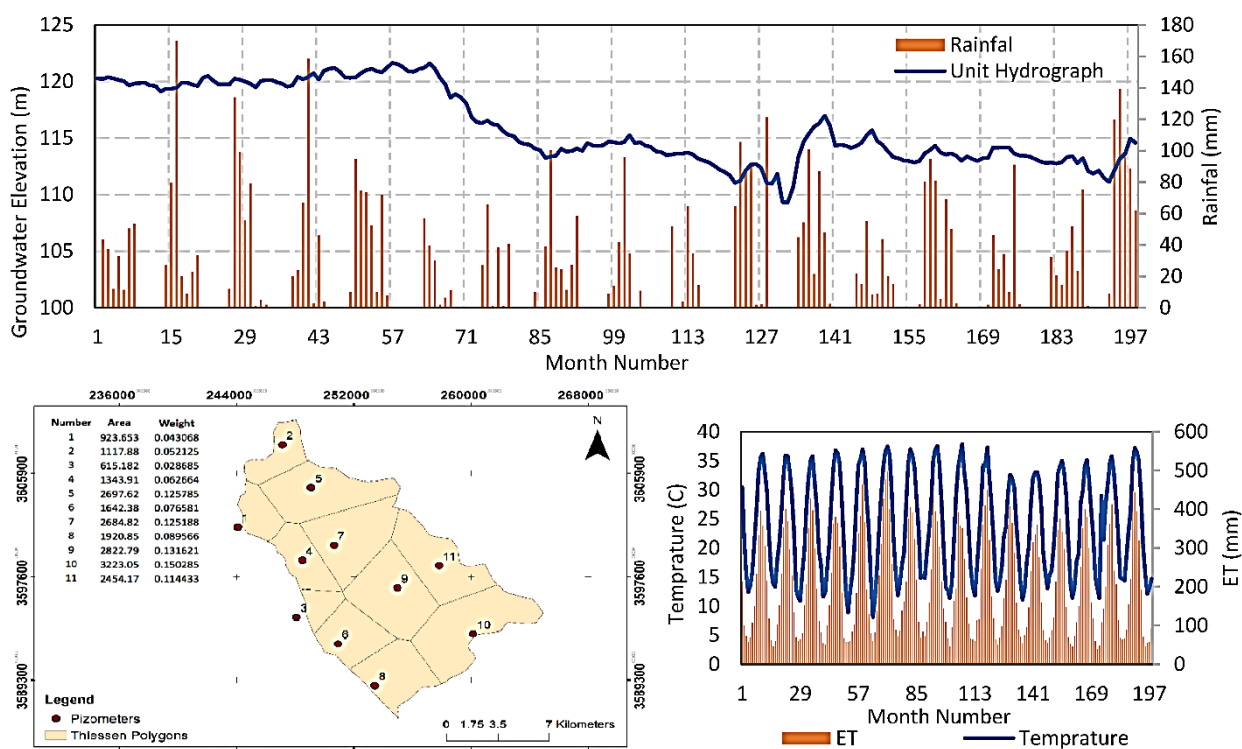
شکل ۷- هیدروگراف واحد آب زیرزمینی (m) و بارندگی (mm) در کل دوره مطالعاتی در دشت ب- پلیگون‌های تیسسن و وزن هر پیزومتر ج- مقادیر دما (C) و تبخیر (mm) در کل دوره مطالعاتی در دشت
