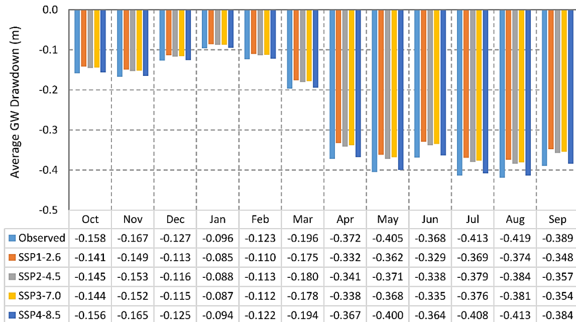
شکل ۹- میانگین بلند مدت تغییرات تراز آبخوان در ماه‌های مختلف در دوره‌ی ۲۰۵۰-۲۰۲۳ و دوره پایه - مدل Hybrid
