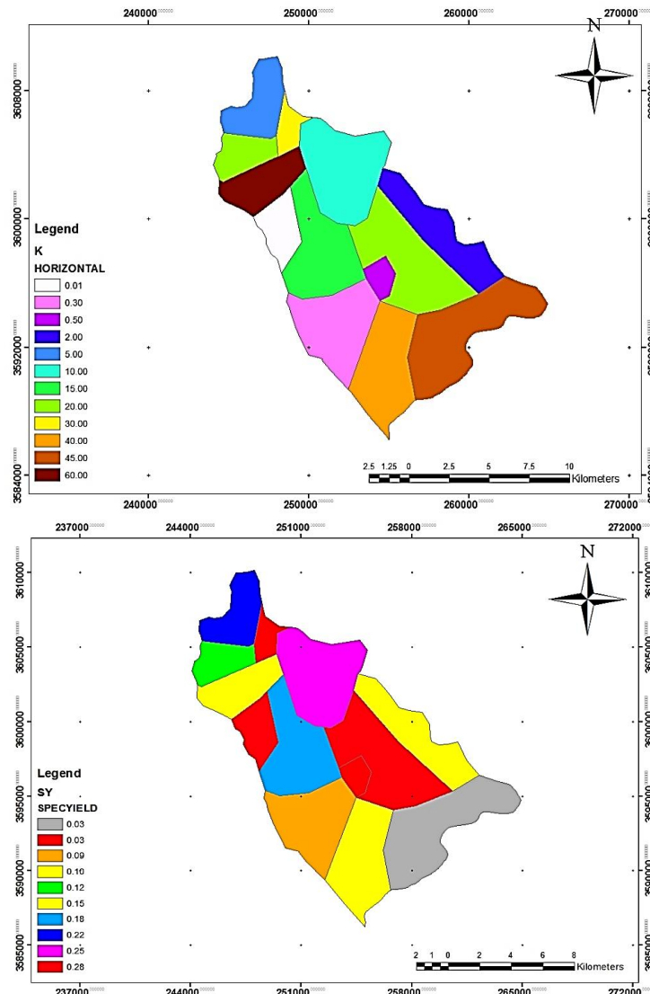
شکل ۶- پهنه بندی مقادیر هدایت هیدرولیکی (متر در روز) و آبدهی ویژه واسنجی شده (اعشاری) در محدوده مطالعاتی
