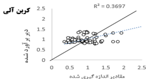
شکل ۳- مقادیر متغیرهای اندازه‌گیری شده در برابر مقادیر برآوردشده آنها با روش‌های مختلف درون‌یابی: پتاسیم، روی و منگنز به روش کریجینگ و فسفر، آهن و مس به روش IDW-1
