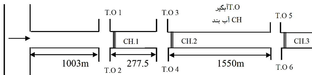
شکل ۱. طرح شماتیک کانال E1R1
