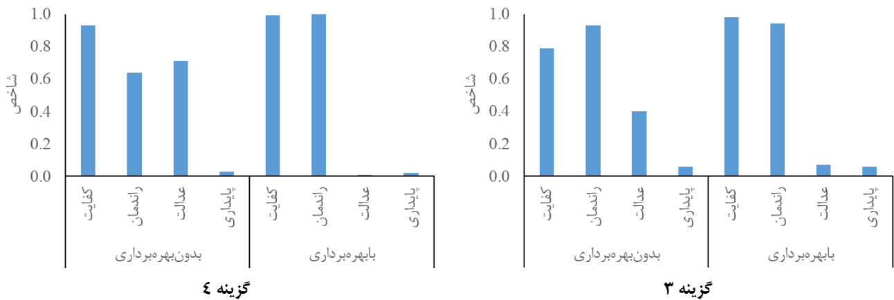
شکل ۴. مقادیر شاخص‌های ارزیابی عملکرد در حالت بهره‌برداری به‌هنگام و باز بودن آبگیرهای ۵ و ۶، گزینه ۳: افزایش دبی و گزینه ۴: کاهش دبی.
