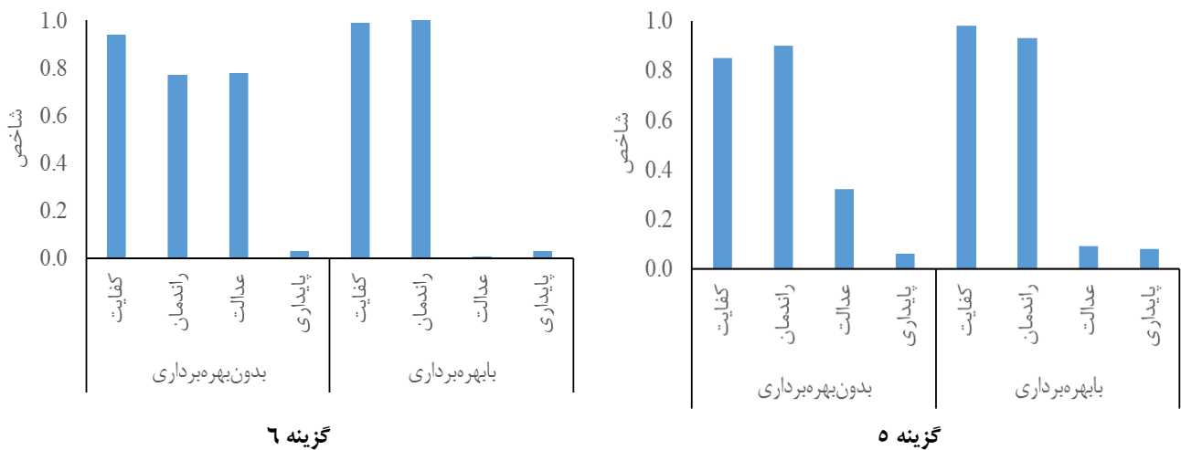
شکل ۵. مقادیر شاخص‌های ارزیابی عملکرد در حالت بهره‌برداری به‌هنگام و باز بودن آبگیرهای ۳ تا ۶، گزینه ۵: افزایش دبی و گزینه ۶: کاهش دبی.
