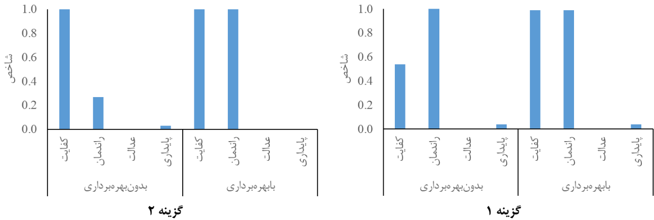
شکل ۳. مقادیر شاخص‌های ارزیابی عملکرد در حالت بهره‌برداری دیر هنگام، گزینه ۱: افزایش دبی و گزینه ۲: کاهش دبی.
