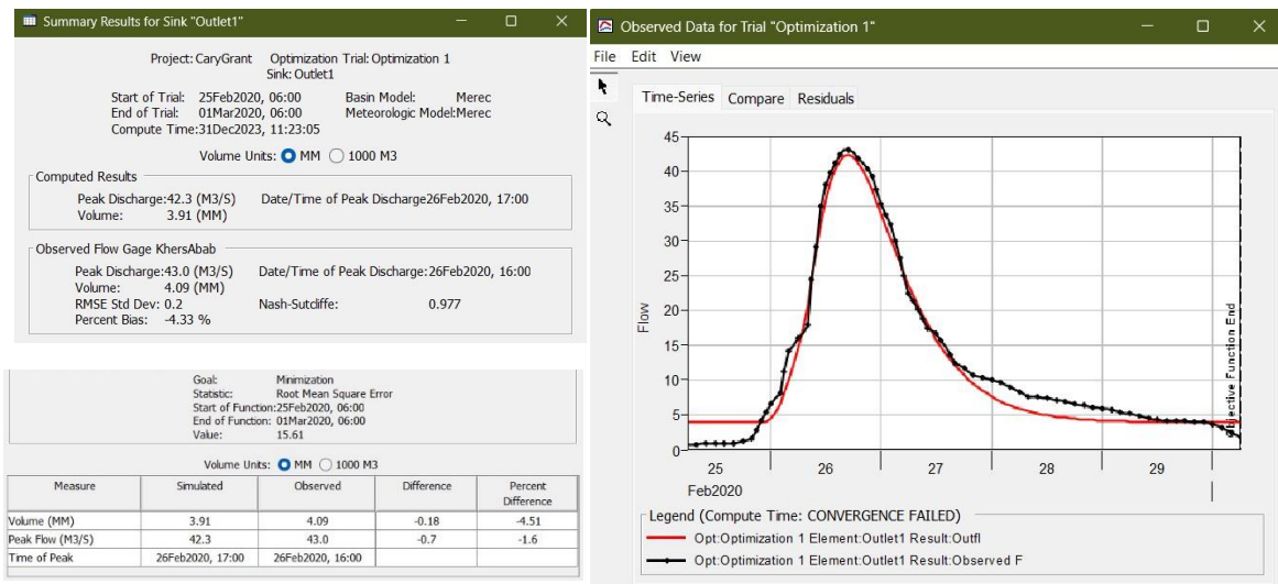
شکل ۶. هیدروگراف و مقادیر دبی پیک و حجم سیلاب
