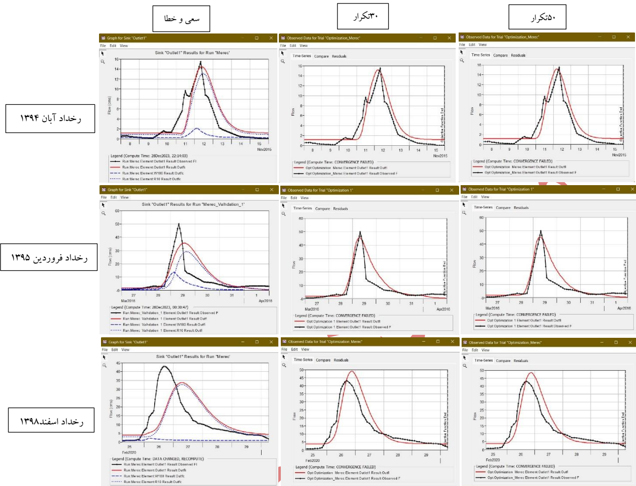
شکل ۵. مقایسه هیدروگراف‌های سه رخداد بعد از بهینه سازی
