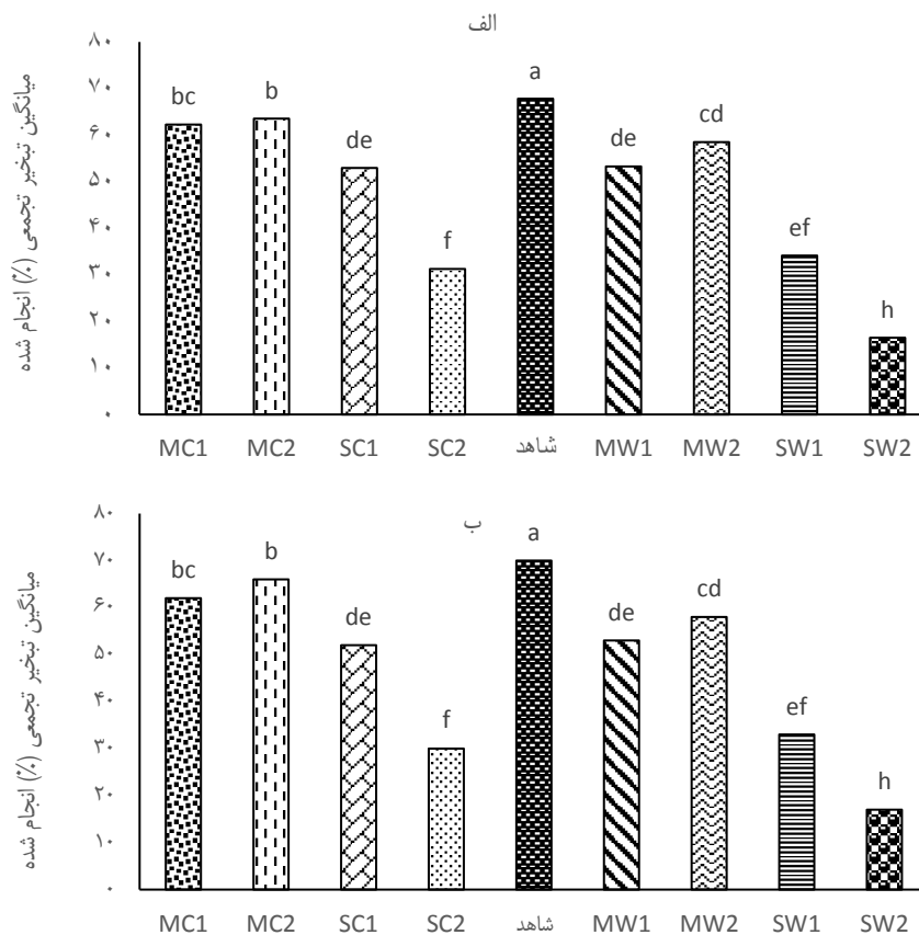
شکل ۱. اثر متقابل نوع، سطوح و نحوه کاربرد مواد اصلاح کننده بر مقدار تبخیر دو دوره الف) ۱۰ روزه و ب) ۱۸ روزه خرداد ماه (M: کاربرد مخلوط، S: کاربرد سطحی، C: کود گاوی، W: کاه و کلش گندم اعداد ۱ و ۲: به ترتیب ۱ و ۵ درصد مواد اصلاحی)
