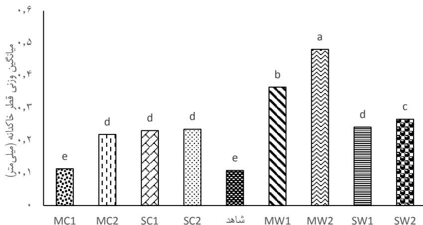
شکل ۳. اثر متقابل نوع، سطوح و نحوه کاربرد مواد اصلاح کننده بر میانگین وزنی قطر خاکدانه‌ها (M: کاربرد مخلوط، S: کاربرد سطحی، C: کود گاوی، W: کاه و کلش گندم اعداد ۱ و ۲: به ترتیب ۱ و ۵ درصد مواد اصلاحی)
