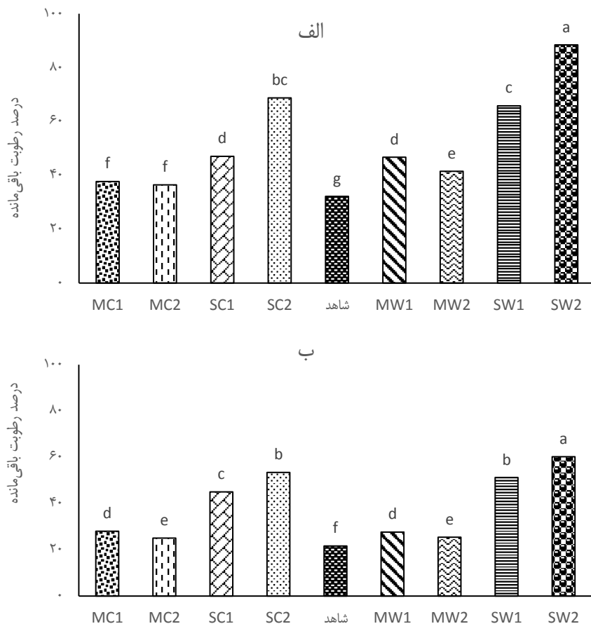
شکل ۳. اثر متقابل نوع، سطوح و نحوه کاربرد مواد اصلاح کننده بر مقدار رطوبت باقی مانده خاک دو دوره الف) خرداد و ب) مرداد ماه (M: کاربرد مخلوط، S: کاربرد سطحی، C: کود گاوی، W: کاه و گلش گندم اعداد ۱ و ۲: به ترتیب ۱ و ۵ درصد مواد اصلاحی)
