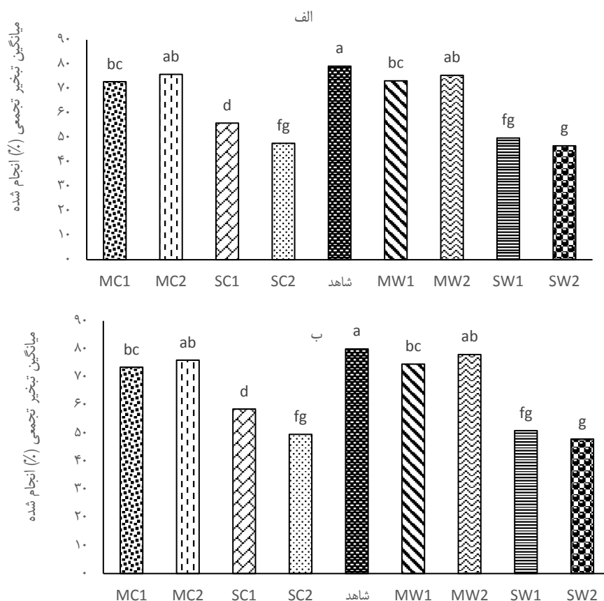
شکل ۲. اثر متقابل نوع، سطوح و نحوه کاربرد مواد اصلاح کننده بر مقدار تبخیر دو دوره الف) ۱۰ روزه و ب) ۱۸ روزه مرداد ماه (M: کاربرد مخلوط، S: کاربرد سطحی، C: کود گاوی، W: کاه و کلش گندم اعداد ۱ و ۲: به ترتیب ۱ و ۵ درصد مواد اصلاحی)
