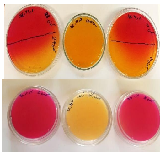
شکل ۱- تغییر رنگ معرف فنل رد در محیط کشت UAB (الف) و در محیط کشت اختصاصی M9 (ب) به ترتیب به دلیل ایجاد محیط قلیایی در نتیجه فعالیت اوره‌آزی ال-آسپاراژینازی جدایه‌ها در کنار نمونه‌های شاهد (بدون مایه‌زنی باکتری) پس از ۲۴ ساعت انکوباسیون
