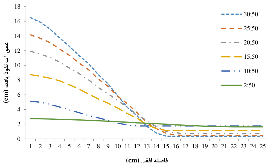
شکل ۵- نفوذ نقطه ای برای عمق های مختلف ساختار کجاوه
