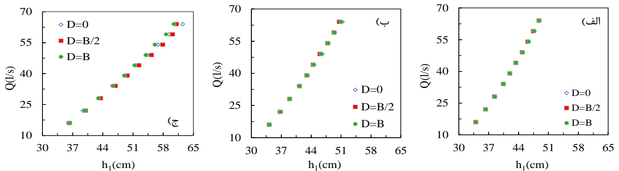
شکل ۸. مقایسه تغییرات دبی-اشل عمق بالادست دریاچه سالونی ( h_1 ) در موقعیت‌های مختلف قرارگیری پارشال فلوم ۱ فوت در شرایط جریان آزاد: (الف) b/B=0.34 , (ب) b/B=0.23 , (ج) b/B=0.11
