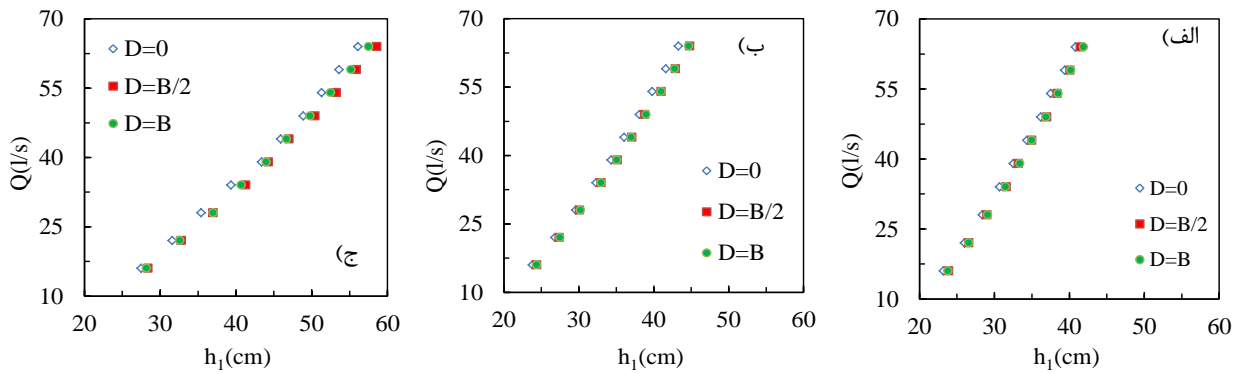
شکل ۷. مقایسه تغییرات دبی-اشل عمق بالادست دریاچه سالونی ( h_1 ) در موقعیت‌های مختلف قرارگیری پارشال فلوم ۹ اینچ در شرایط جریان آزاد: (الف) b/B=0.34 , (ب) b/B=0.23 , (ج) b/B=0.11
