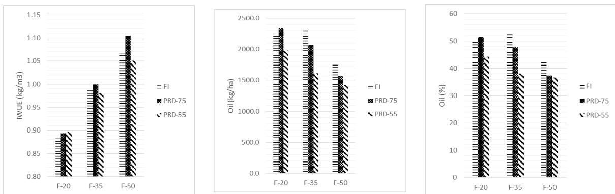
شکل ۵. به ترتیب از راست به چپ نمودارهای درصد روغن، عملکرد روغن و کارایی مصرف آب آبیاری برای ۹ حالت مختلف دور آبیاری و مقدار آب آبیاری در
