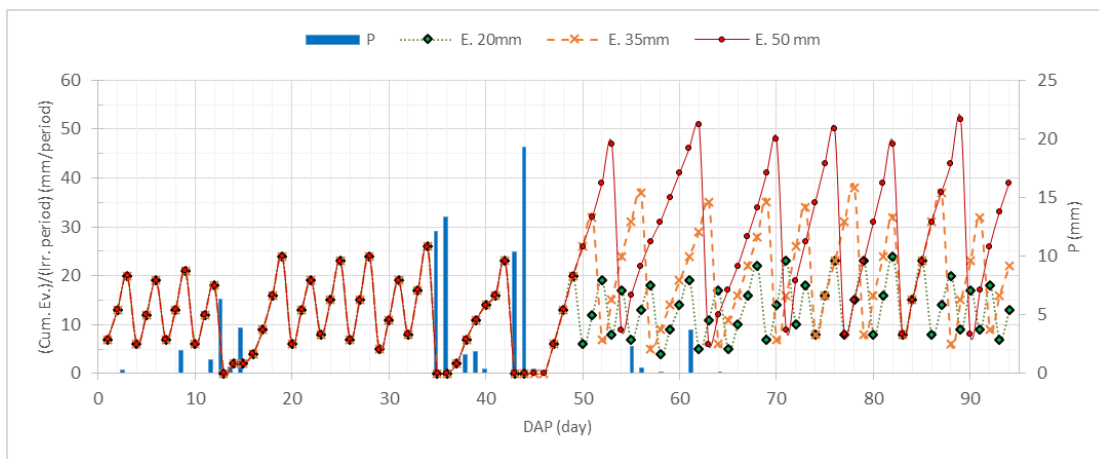
شکل ۴. تبخیر تجمعی از تشت تبخیر کلاس A سال ۱۳۹۵ به منظور تعیین زمان انجام آبیاری برای دورهای آبیاری مختلف (DAP: روز بعد از کاشت (روز)، (Cum. Ev.)/(Irr. period): تبخیر تجمعی در دور آبیاری (میلی‌متر در دور آبیاری و P: بارندگی (میلی‌متر))
