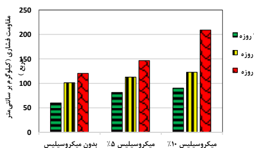
شکل ۱۲- مقاومت فشاری نمونه‌ها در ۱۲٪ سیمان
