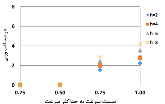
شکل ۱۸- درصد افت وزنی نمونهها در ۳۰٪ سیمان، \Theta=30^\circ
