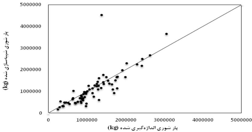
شکل ۷- همبستگی بین داده‌های شبیه‌سازی و اندازه‌گیری شده بار شوری در کل حوضه آبریز ناورود در مرحله اعتبارسنجی تحت چرخه نیتروژن
