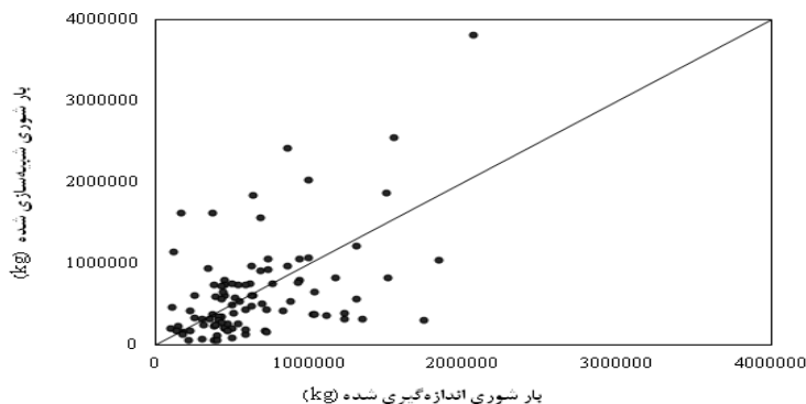
شکل ۸- همبستگی بین داده‌های شبیه‌سازی و اندازه‌گیری شده بار شوری در ایستگاه خلیان حوضه آبریز ناورود تحت چرخه فلزات سنگین در مدل SWAT
