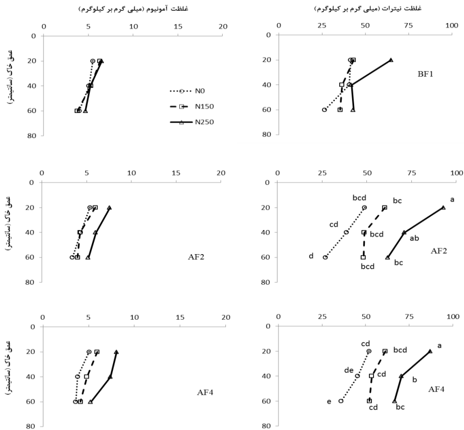
شکل ۵. توزیع غلظت نیترات و آمونیوم در زیر پشته در سه مرحله نمونه برداری (BF1: یک روز قبل از کود دهی، AF2: دو روز بعد از کود دهی، AF4: چهار روز بعد از کود دهی) در تیمارهای مختلف. (مقایسه میانگین به روش توکی در سطح معنی داری ۵ درصد انجام شده است).
