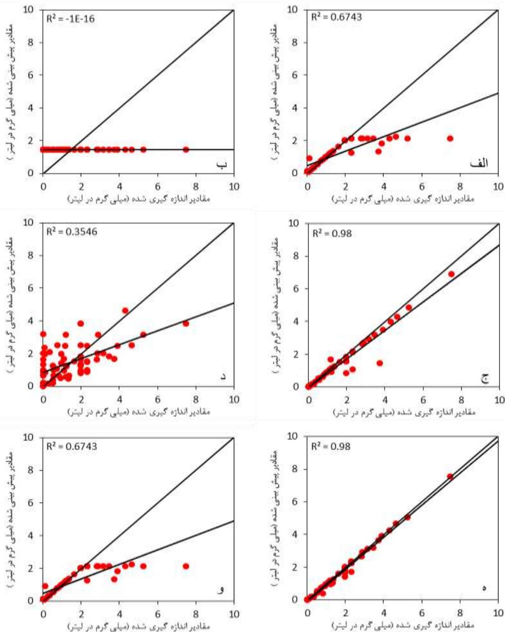
شکل ۴. نمودار پراکندگی مقادیر مشاهده‌شده و پیش‌بینی‌شده رسوب حداقل توسط مدل‌های الف: شبکه عصبی مصنوعی، ب: رگرسیون خطی، ج: فرآیند گوسی، د: k نزدیک‌ترین همسایه، ه: ماشین بردار پشتیبان تکاملی و و: ماشین بردار پشتیبان
