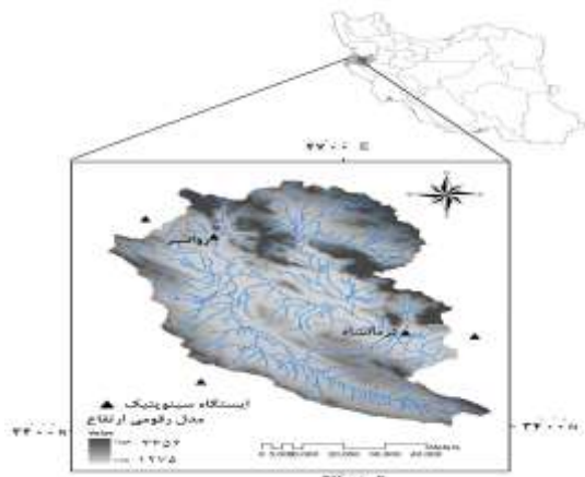
شکل ۱. نمای از موقعیت ایستگاه‌های سینوپتیک کرمانشاه و روانسر
