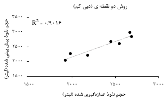
شکل ۱- مقایسه مقادیر اندازه‌گیری شده و پیش‌بینی شده حجم آب نفوذ یافته توسط روش‌های مختلف
