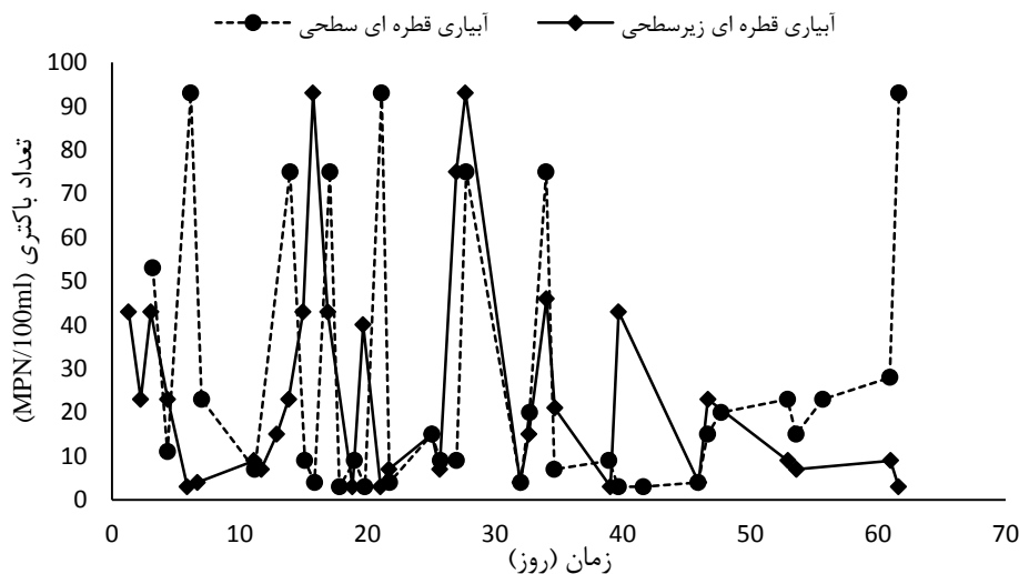
شکل ۹. تعداد باکتری در زهاب خروجی آبیاری قطره‌ای زیرسطحی و سطحی
